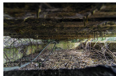
Depuis la tour d'observation, vue intérieure du double couverture de la partie est de l'édifice, servant de chambre d'explosion Phot. Jean-Marc Ramette IVR32_20165901142NUCA
