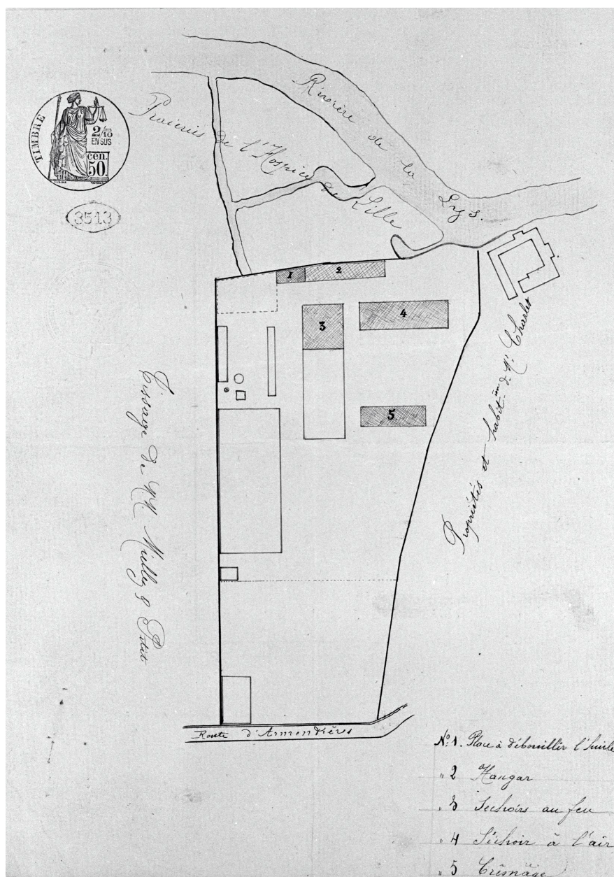
Delattre-Camblain, plan masse, 1875 (AD Nord ; M4173687).
