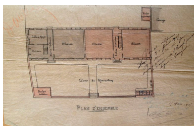
Plan du rez-de-chaussée par Anatole Bienaimé, 1903 (AD Somme ; 99 O 680). Phot. Fournier Bertrand (reproduction) IVR22_20088015017NUCA
