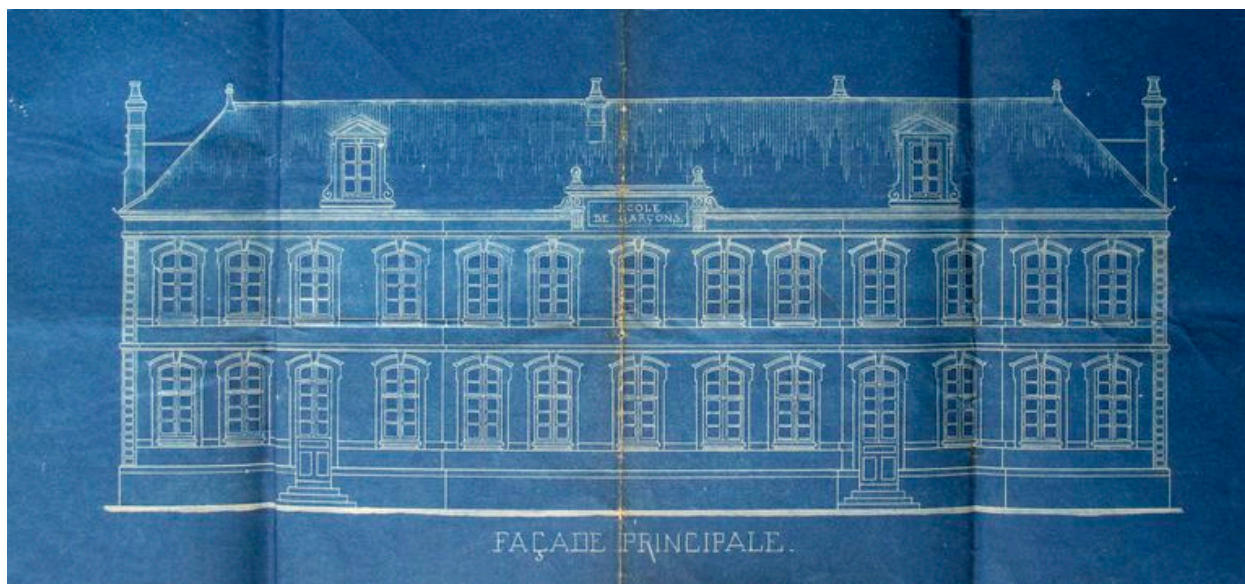
Façade par Anatole Bienaimé, 1903 (AD Somme ; 99 O 680).
