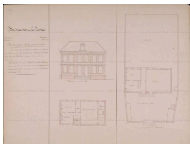
Berteaucourt-les-Dames. Plan de la nouvelle maison d'école de garçons et mairie, 1878 (AD Somme ; 99 T 3804 94/2). Phot. Archives départementales de la Somme (reproduction) IVR22_20138016162NUC2A
