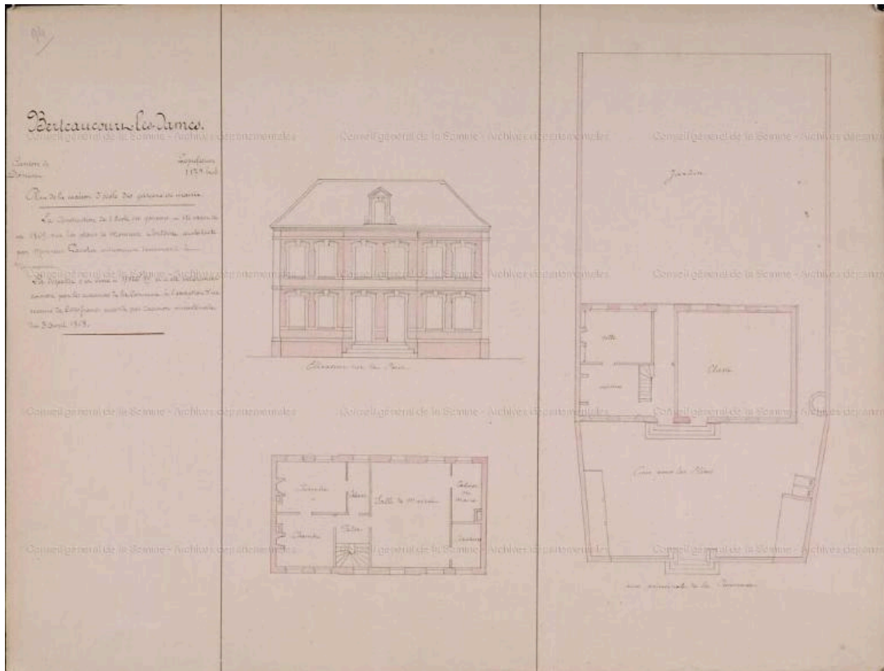
Berteaucourt-les-Dames. Plan de la nouvelle maison d'école de garçons et mairie, 1878 (AD Somme ; 99 T 3804 94/2).
