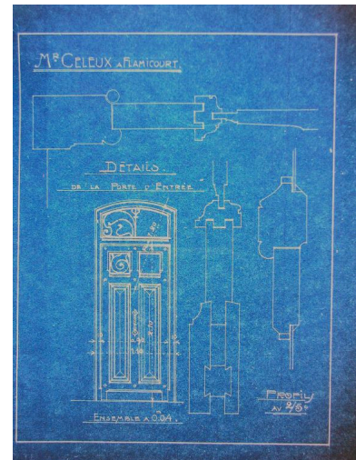
Détail de la porte d'entrée, A. Castex (architecte), vers 1920 (AD Somme ; 10 R 407).
