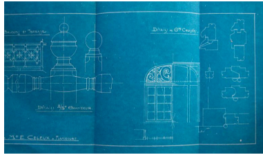
Détails, menuiseries des fenêtres, balcons et terrasse, A. Castex (architecte), vers 1920 (AD Somme ; 10 R 407). Phot. Gilles-Henri Bailly IVR22_20158005543NUCA
