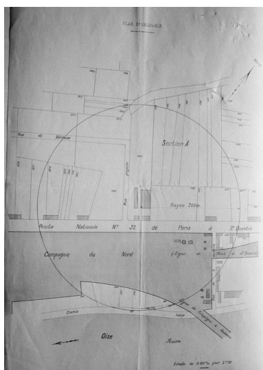
Plan masse d'ensemble pour l'implantation de la brosserie
