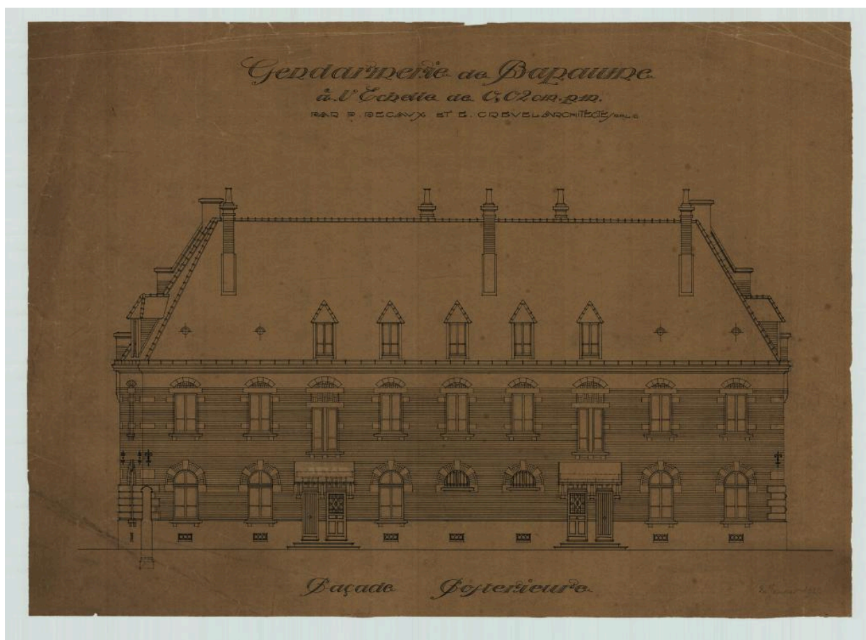
Gendarmerie de Bapaume. Dessin de la façade postérieure. Signé P. Decaux et É. Crevel, architectes, 20 janvier 1923. (AD Pas-de-Calais, 4N0658).
