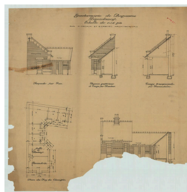
Gendarmerie de Bapaume. Dépendances : façade sur rue ; pignon postérieur et coupe sur bûcherie ; coupe transversale sur buanderie ; plan du rez-de-chaussée ; façade sur cour. Signé P. Decaux et É. Crevel, architectes. Sans date (manque). (AD Pas-de-Calais, 4N0684) Phot. Pierre Thibaut IVR32_20216200862NUCA
