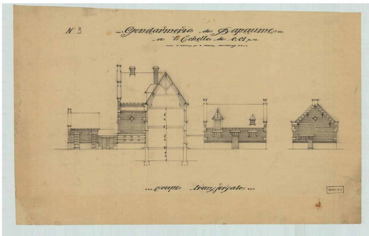
Gendarmerie de Bapaume. Coupe transversale. Signé P. Decaux et É. Crevel, architectes, 18 février 1922. (AD Pas-de-Calais, 4N0652)
