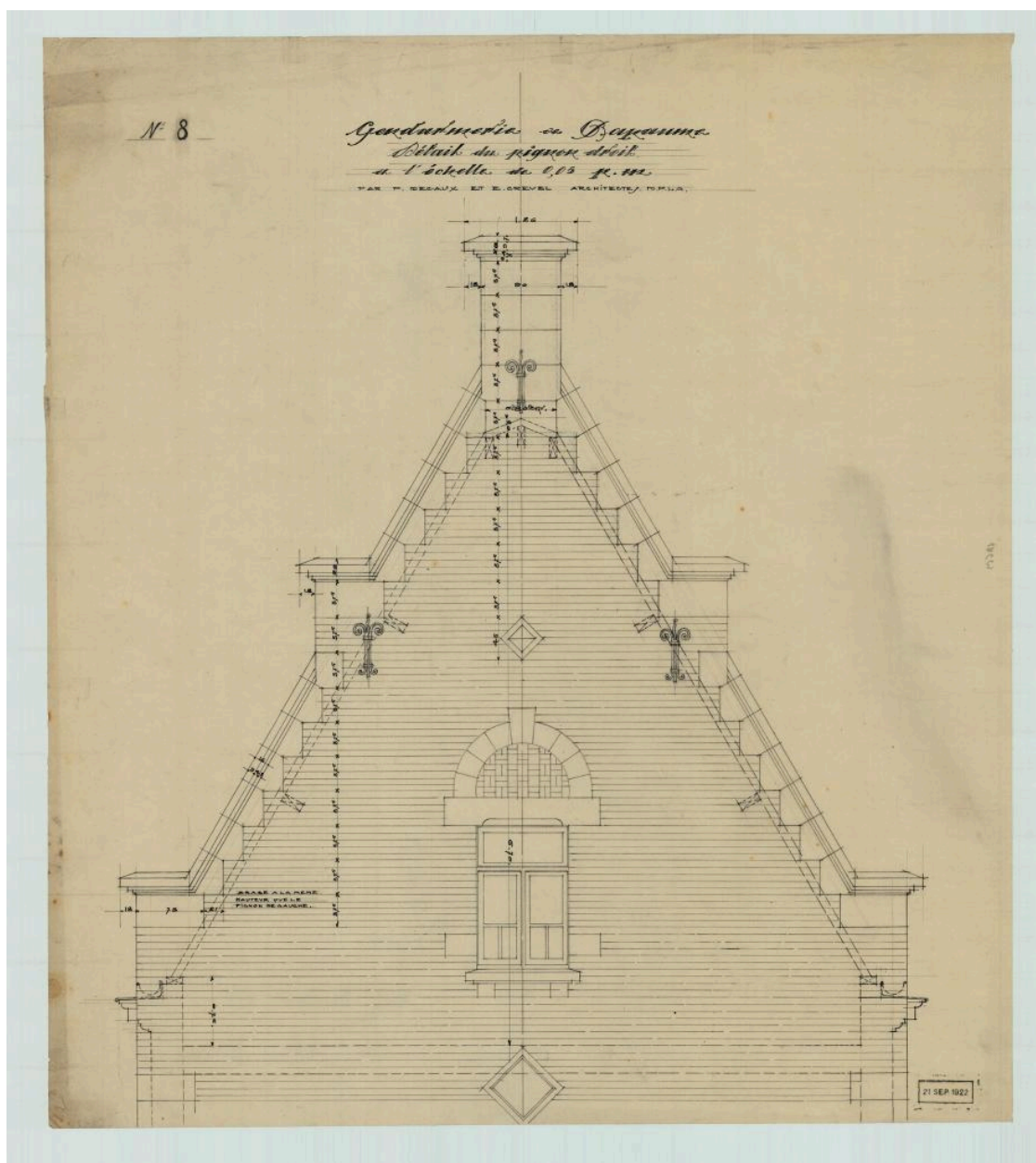
Gendarmerie de Bapaume. Dessin d'un pignon de la façade principale. Signé P. Decaux et É. Crevel, architectes, 21 septembre 1922. (AD Pas-de-Calais, 4N0669)
