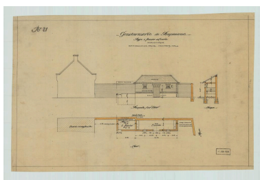
Gendarmerie de Bapaume. Fosse à fumier et écurie : façade sur cour, plan. Signé P. Decaux et É. Crevel, architectes, 1er juin 1923. (AD Pas-de-Calais, 4N0682) Phot. Pierre Thibaut IVR32_20216200861NUCA
