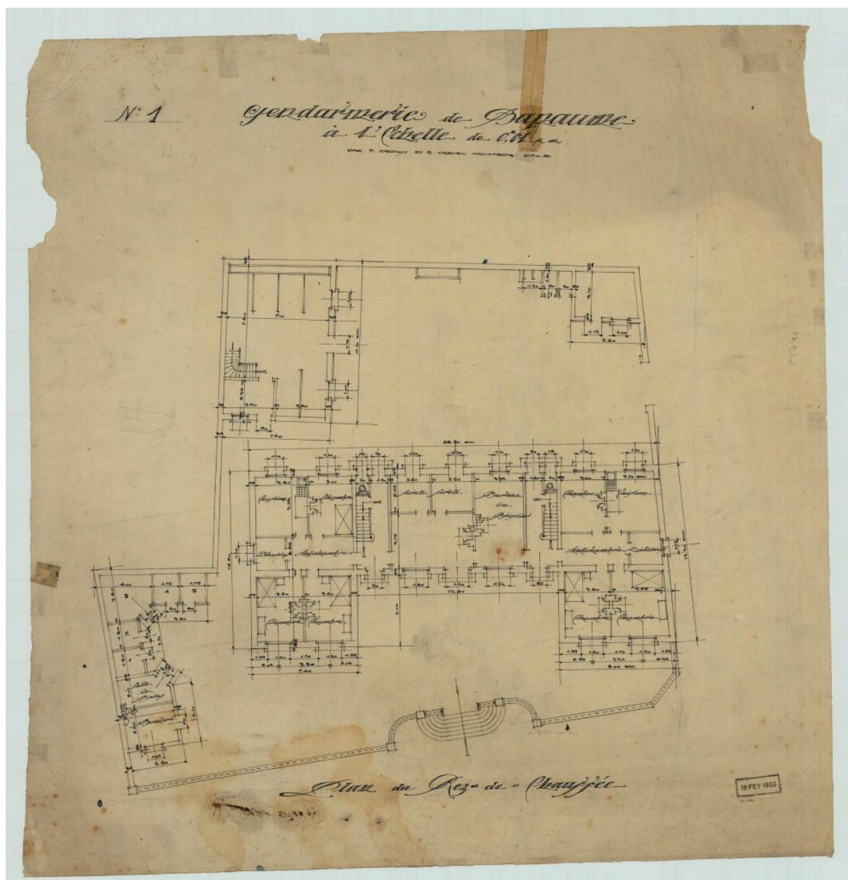
Gendarmerie de Bapaume. Plan du rez-de-chaussée. Signé P. Decaux et É. Crevel, architectes, 18 février 1922. (AD Pas-de-Calais, 4N0659)
