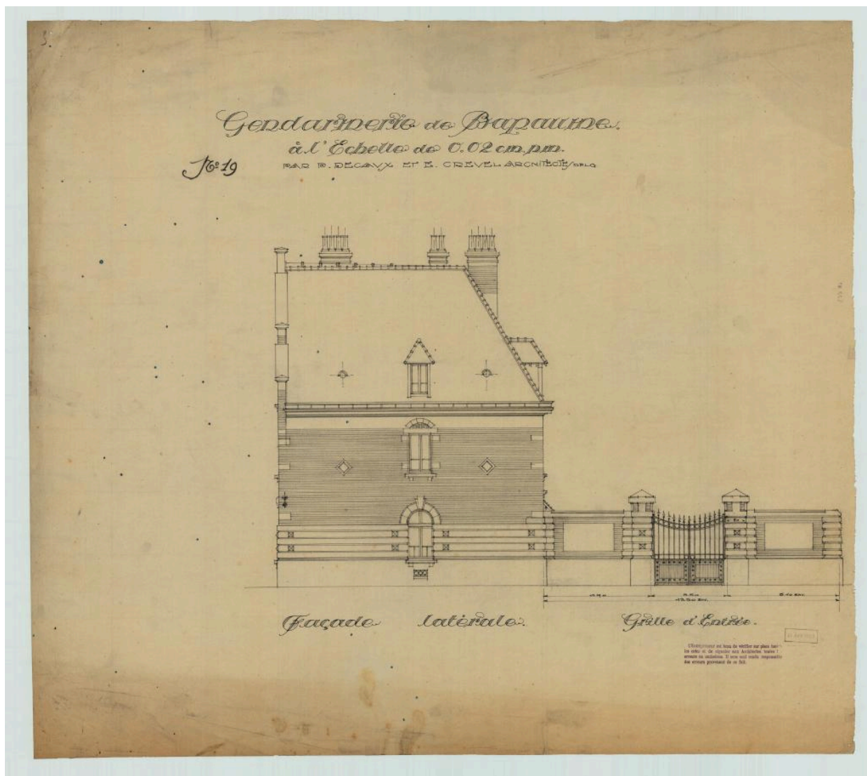
Gendarmerie de Bapaume. Dessin de la façade latérale et de la grille d'entrée. Signé P. Decaux et É. Crevel, architectes, 21 avril 1923. (AD Pas-de-Calais, 4N0663)
