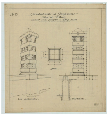
Gendarmerie de Bapaume. Détail d'un pilastre : vue perspective, plan, élévation. Signé P. Decaux et É. Crevel, architectes, 28 juin 1923. (AD Pas-de-Calais, 4N0672) Phot. Pierre Thibaut IVR32_20216200857NUCA
