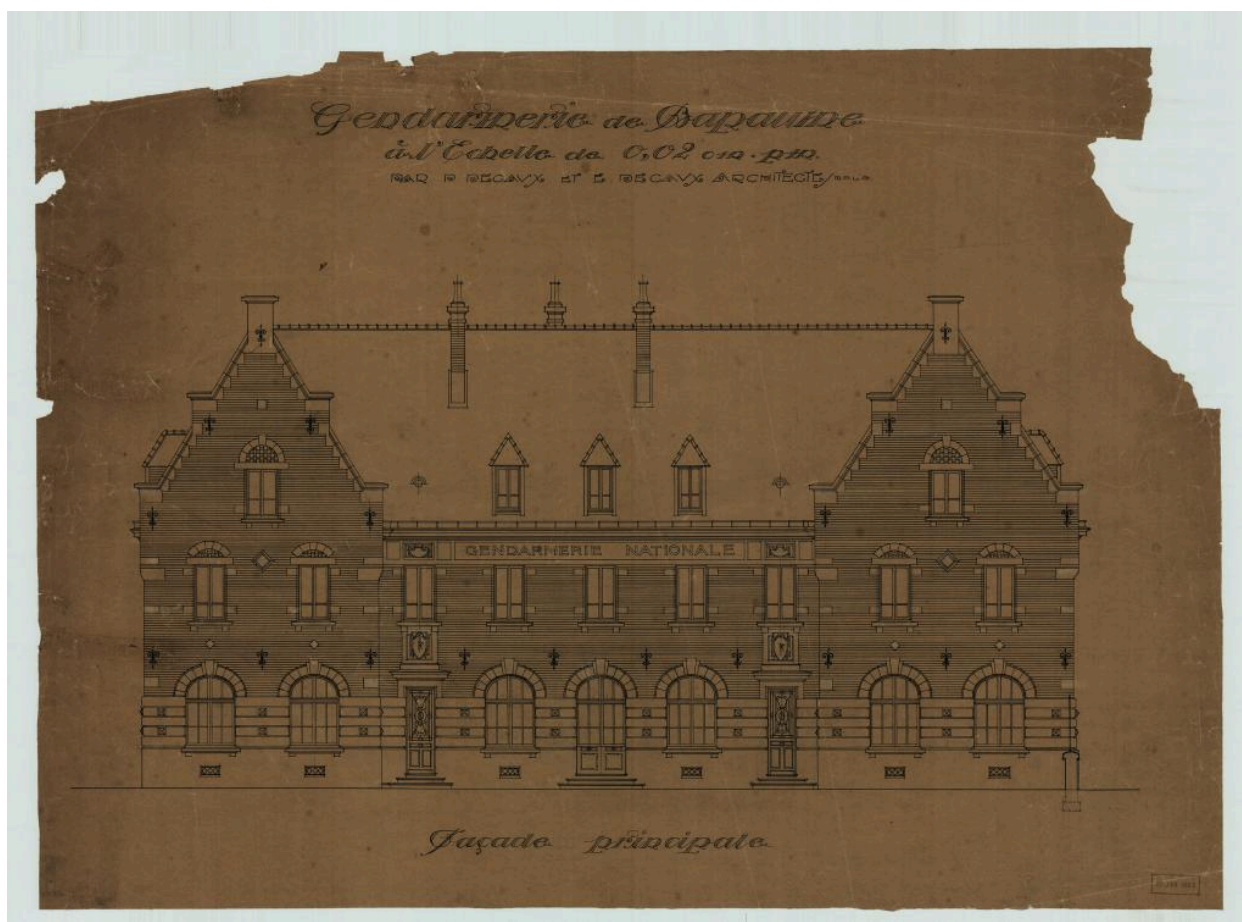
Gendarmerie de Bapaume. Dessin de la façade principale. Signé P. Decaux et É. Crevel, architectes, 20 janvier 1923. (AD Pas-de-Calais, 4N0651)
