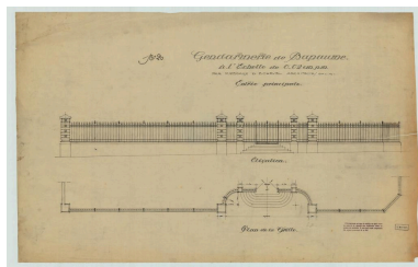
Gendarmerie de Bapaume. Entrée principale : élévation, plan de la grille. Signé P. Decaux et É. Crevel, architectes, 12 mai 1923. (AD Pas-de-Calais, 4N0676) Phot. Pierre Thibaut IVR32_20216200858NUCA
