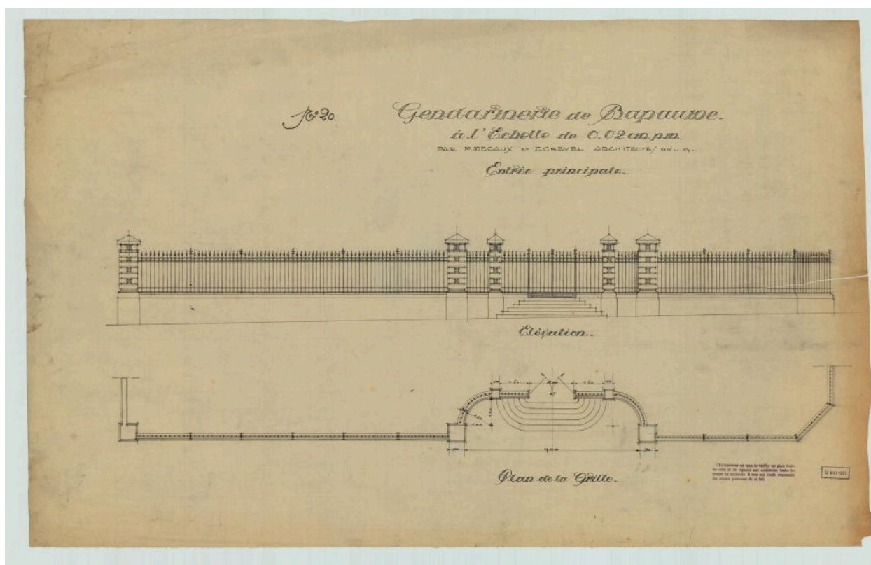
Gendarmerie de Bapaume. Entrée principale : élévation, plan de la grille. Signé P. Decaux et É. Crevel, architectes, 12 mai 1923. (AD Pas-de-Calais, 4N0676)
