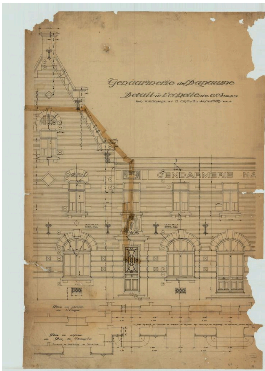
Gendarmerie de Bapaume. Dessin d'un détail de la façade principale. Signé P. Decaux et É. Crevel, architectes, 20 janvier 1923. (AD Pas-de-Calais, 4N0662) Le plan précise les hauteurs des reliefs des différents éléments décoratifs de la façade.
