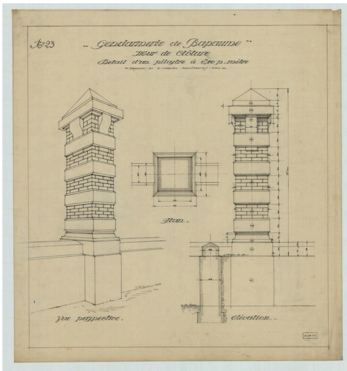
Gendarmerie de Bapaume. Détail d'un pilastre : vue perspective, plan, élévation. Signé P. Decaux et É. Crevel, architectes, 28 juin 1923. (AD Pas-de-Calais, 4N0672)
