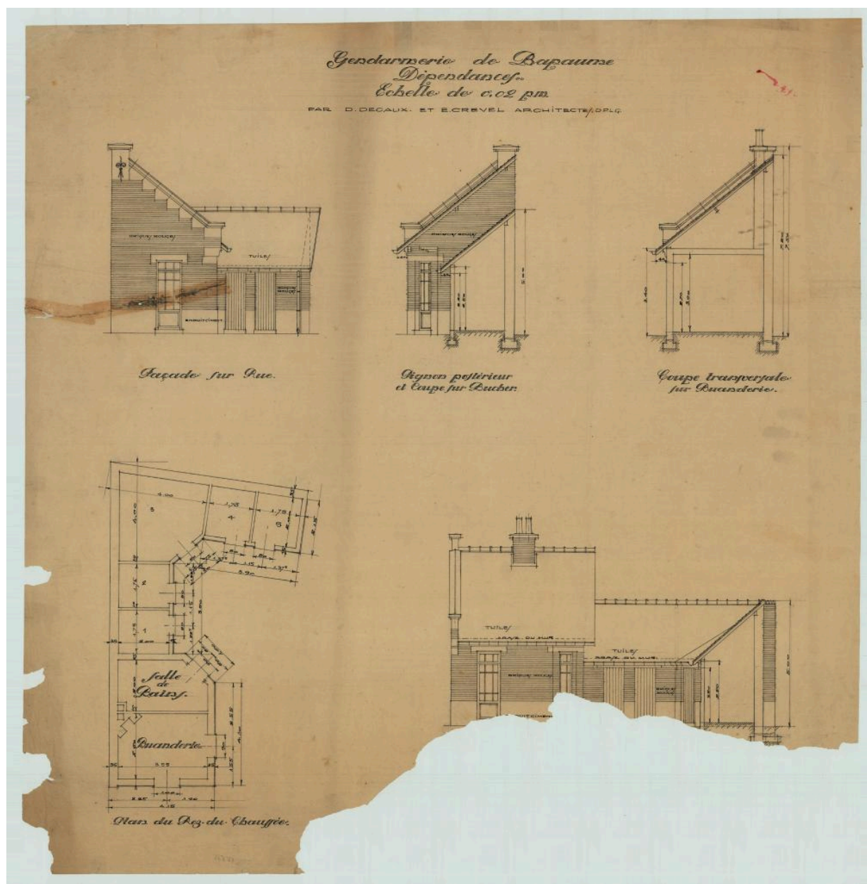
Gendarmerie de Bapaume. Dépendances : façade sur rue ; pignon postérieur et coupe sur bûcher ; coupe transversale sur buanderie ; plan du rez-de-chaussée ; façade sur cour. Signé P. Decaux et É. Crevel, architectes. Sans date (manque). (AD Pas-de-Calais, 4N0684)
