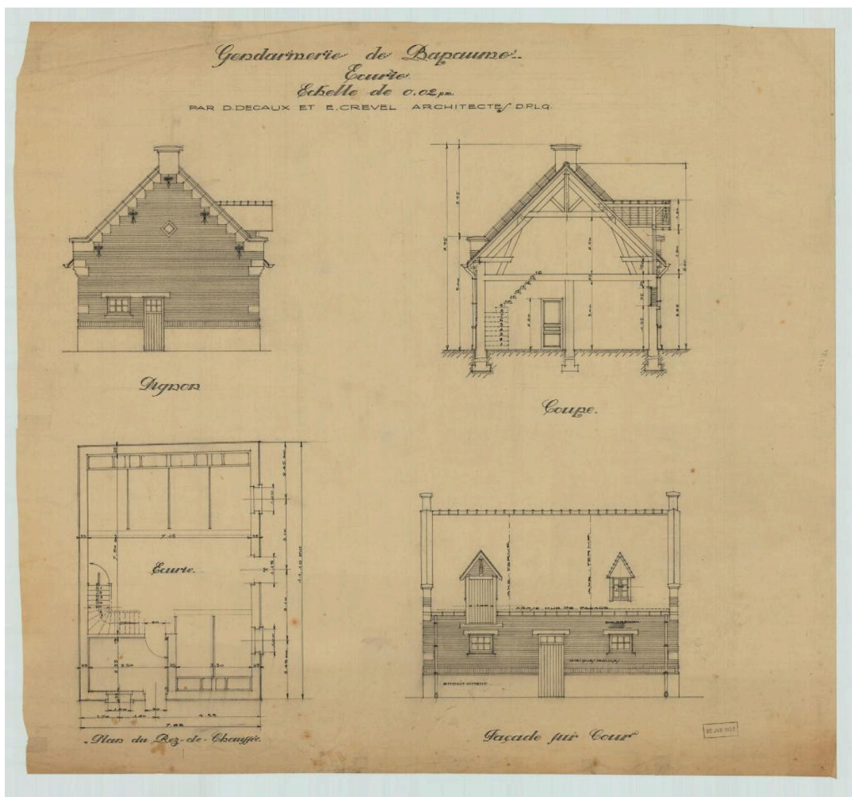
Gendarmerie de Bapaume. Écurie, pignon, coupe, plan du rez-de-chaussée, façade sur cour. Signé P. Decaux et É. Crevel, architectes, 20 janvier 1923. (AD Pas-de-Calais, 4N0666)
