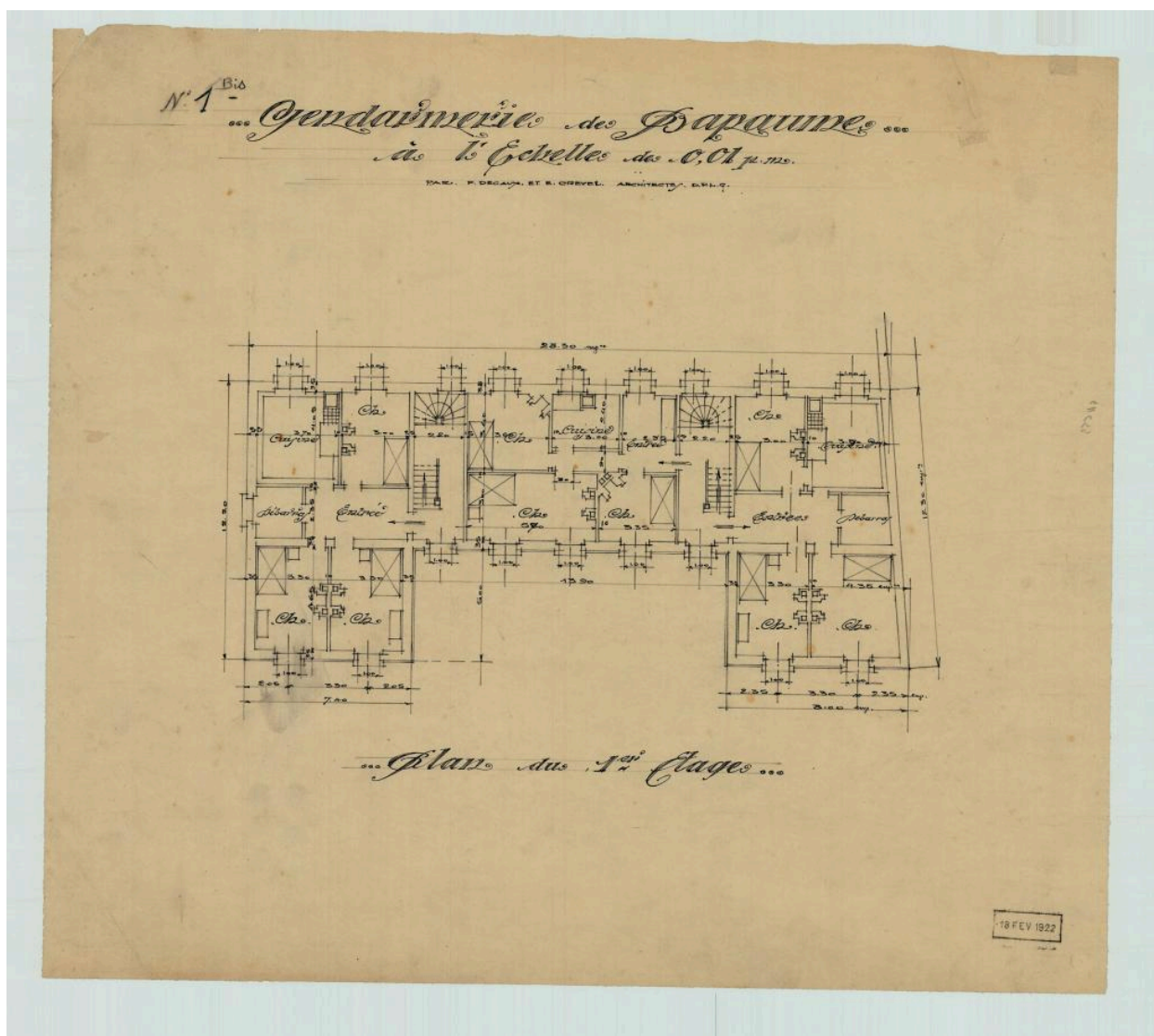
Gendarmerie de Bapaume. Plan du premier étage. Signé P. Decaux et É. Crevel, architectes, 18 février 1922. (AD Pas-de-Calais, 4N0653)
