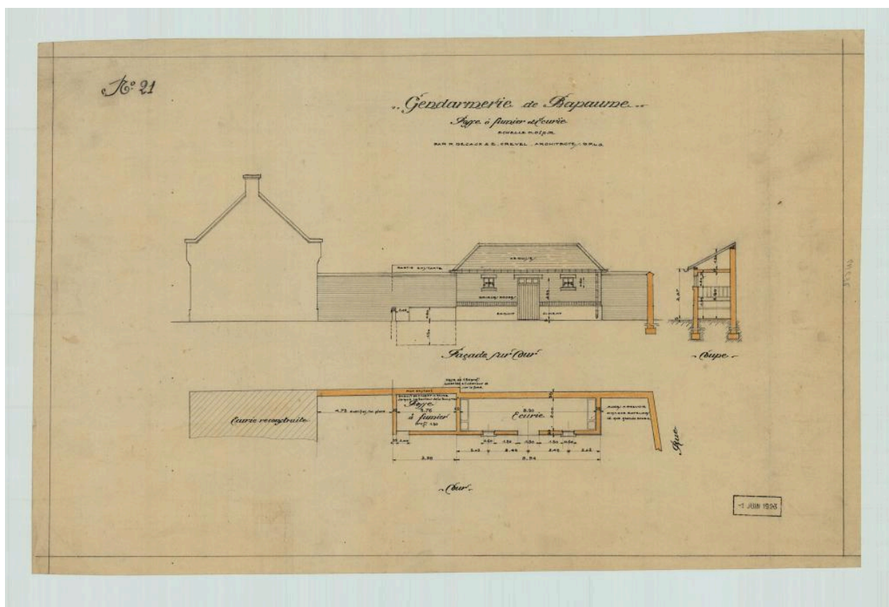
Gendarmerie de Bapaume. Fosse à fumier et écurie : façade sur cour, plan. Signé P. Decaux et É. Crevel, architectes, 1er juin 1923. (AD Pas-de-Calais, 4N0682)
