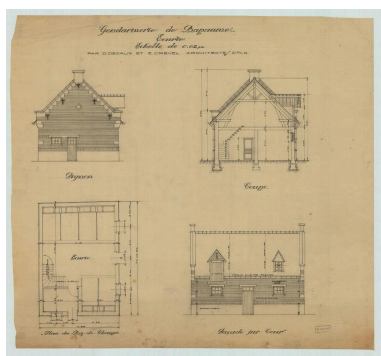
Gendarmerie de Bapaume. Écurie, pignon, coupe, plan du rez-de-chaussée, façade sur cour. Signé P. Decaux et É. Crevel, architectes, 20 janvier 1923. (AD Pas-de-Calais, 4N0666) Phot. Pierre Thibaut IVR32_20216200855NUCA
