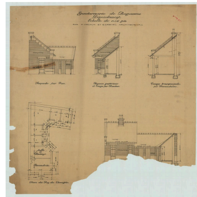
Gendarmerie de Bapaume. Dépendances : façade sur rue ; pignon postérieur et coupe sur bûcherie ; coupe transversale sur buanderie ; plan du rez-de-chaussée ; façade sur cour. Signé P. Decaux et É. Crevel, architectes. Sans date (manque). (AD Pas-de-Calais, 4N0684) Phot. Pierre Thibaut IVR32_20216200862NUCA
