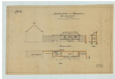
Gendarmerie de Bapaume. Fosse à fumier et écurie : façade sur cour, plan. Signé P. Decaux et É. Crevel, architectes, 1er juin 1923. (AD Pas-de-Calais, 4N0682) Phot. Pierre Thibaut IVR32_20216200861NUCA
