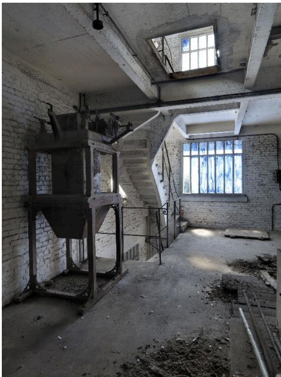
Escalier en béton armé du 2e étage, vue de trois-quarts.
