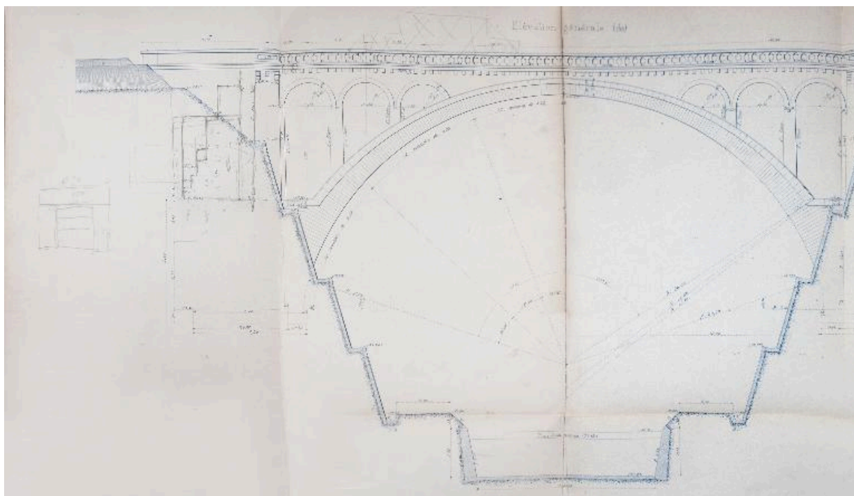
Coupe du projet de l'ouvrage d'art. 1907.
