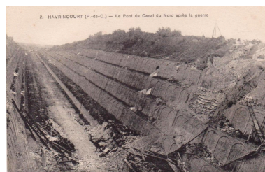
État de la grande tranchée d'Havrincourt après la Première Guerre mondiale. Destruction des ponts et d'une partie des berges maçonnées. Cuvette partiellement comblée. Carte postale, après 1918. Repro. Pierre Thibaut IVR32_20226200278NUCAB
