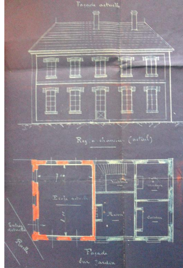
Plan des modifications apportées en 1931 (AD Somme 99 O 1886). Phot. Frédéric-Nicolas Kocourek (reproduction) IVR22_20148005015NUC2A
