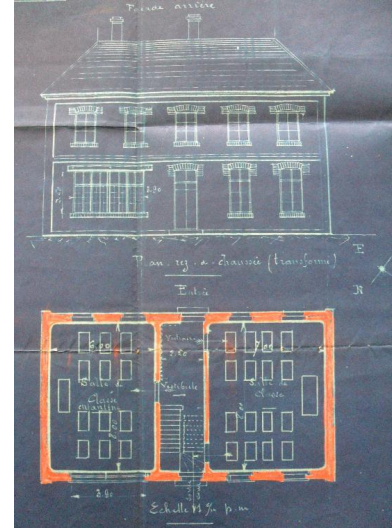
Plan des modifications apportées en 1931 (AD Somme 99 O 1886). Phot. Frédéric-Nicolas Kocourek IVR22_20148005016NUC2A
