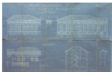
Elévations et coupe de la maison de commerce du tissage Léon, 1920 (BM Saint-Quentin).
