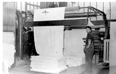
Gratteuse à 24 travailleurs, photographie, 1957 (coll. part.). Repro. Philippot Jacques IVR22_19878000279XB
