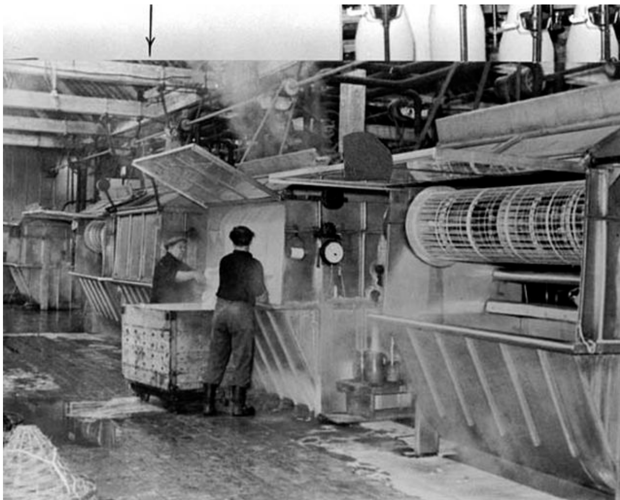
Vue intérieure de l'atelier et des bacs de blanchiment, photographie, 1957 (coll. part.).
