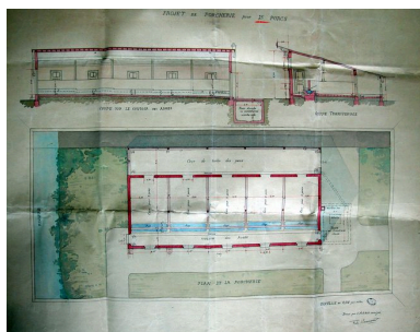
Plan et coupe d'un projet de porcherie pour la laiterie, par Félix Besencenet (architecte), mai 1903. Phot. Fournier Bertrand (reproduction) IVR22_20036000519NUCAB
