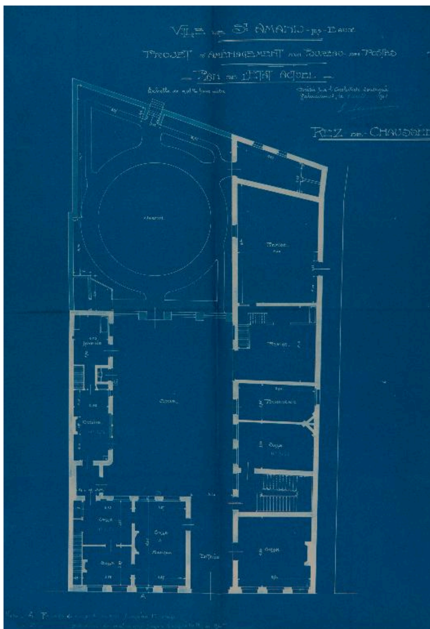
Projet d'aménagement d'un immeuble en bureau de poste ; plan du rez-de-chaussée, Edmond Lemaire architecte, 1911 (AD Nord, 2O 525/146).
