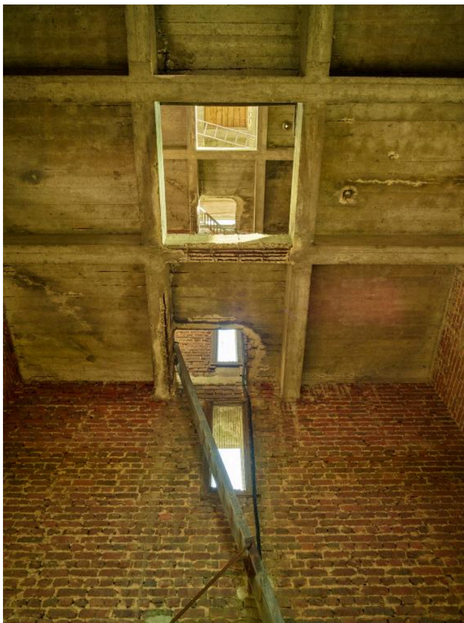
Planchers en béton armé du clocher.
