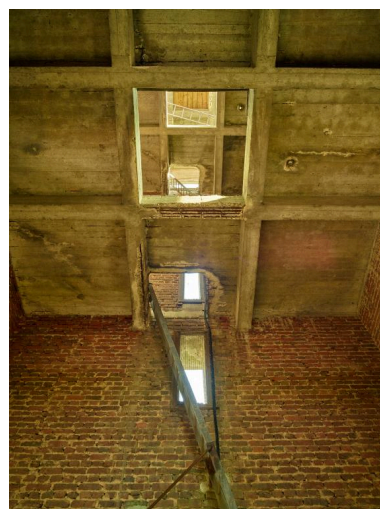
Planchers en béton armé du clocher. Phot. Pierre Thibaut IVR32_20196200070NUCA
