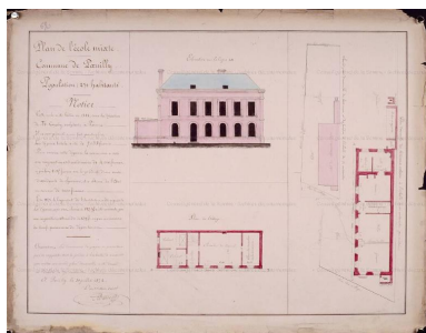
Plan de l'école mixte et de la mairie (AD Somme ; 99 T 3807 630)
