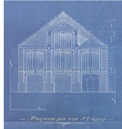
Coupes et élévations, par Jarlat et Grisel, état de 1914 : façade de l'ancienne fonderie, rue Jacques-Lescot (AD Aisne).
