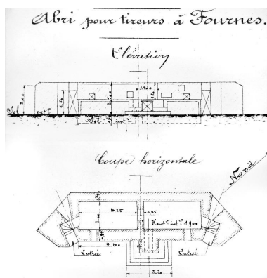
Élévation et coupe horizontale de "l'abri pour tireur" réalisées en juin 1921 par l'architecte des Monuments Historiques. Phot. Jean-Marc Ramette IVR32_20175900386NUCA
