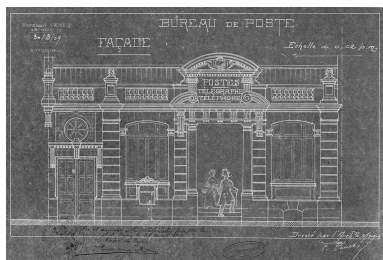
Elévation antérieure, par Venet, 1909 (AD Oise ; série O). Phot. Jean-Michel Périn IVR22_19846000347XB
