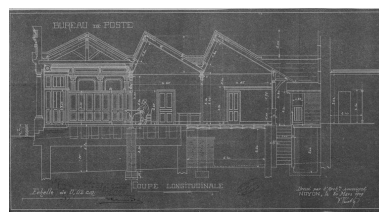
Coupe longitudinale, par Venet, 1909 (AD Oise ; série O). Phot. Jean-Michel Périn IVR22_19846000346XB
