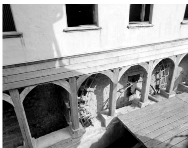
Coursier et roue hydraulique. Phot. Thierry Lefébure IVR22_19908001840X
