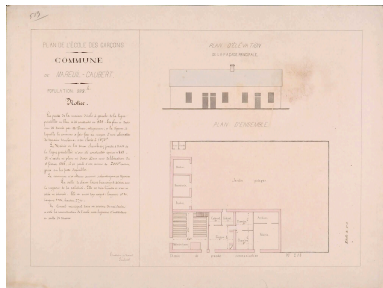
Plan de l'école des garçons, commune de Mareuil-Caubert, 1878. (AD Somme ; 99 T 3806/513_1). Repro. Archives départementales de la Somme IVR32_20238005414NUCA
