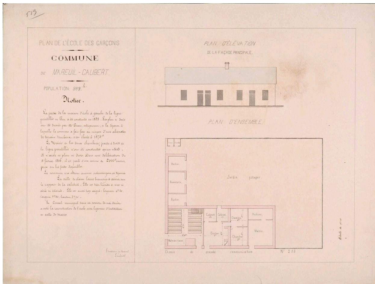
Plan de l'école des garçons, commune de Mareuil-Caubert, 1878. (AD Somme ; 99 T 3806/513_1).
