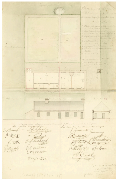
Plan, coupe et élévation de l'école primaire de Zuytpeene avec indications de quelques améliorations, 1840 (AD Nord). Repro. Delphine Volto Jourdan IVR32_20255900054NUCA
