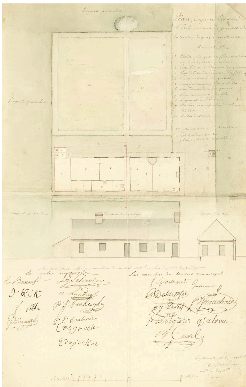
Plan, coupe et élévation de l'école primaire de Zuytpeene avec indications de quelques améliorations, 1840 (AD Nord).
