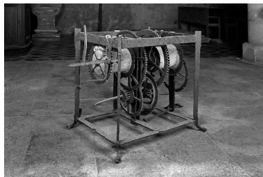
Le mécanisme, vu de trois-quarts.
