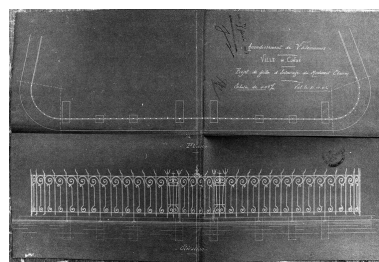
Projet de grille de clôture (non retenu), plan et élévation partiels, 1902 (AD Nord). Repro. Thierry Petitberghien, Autr. Edmond Lemaire IVR31_20025900927X
