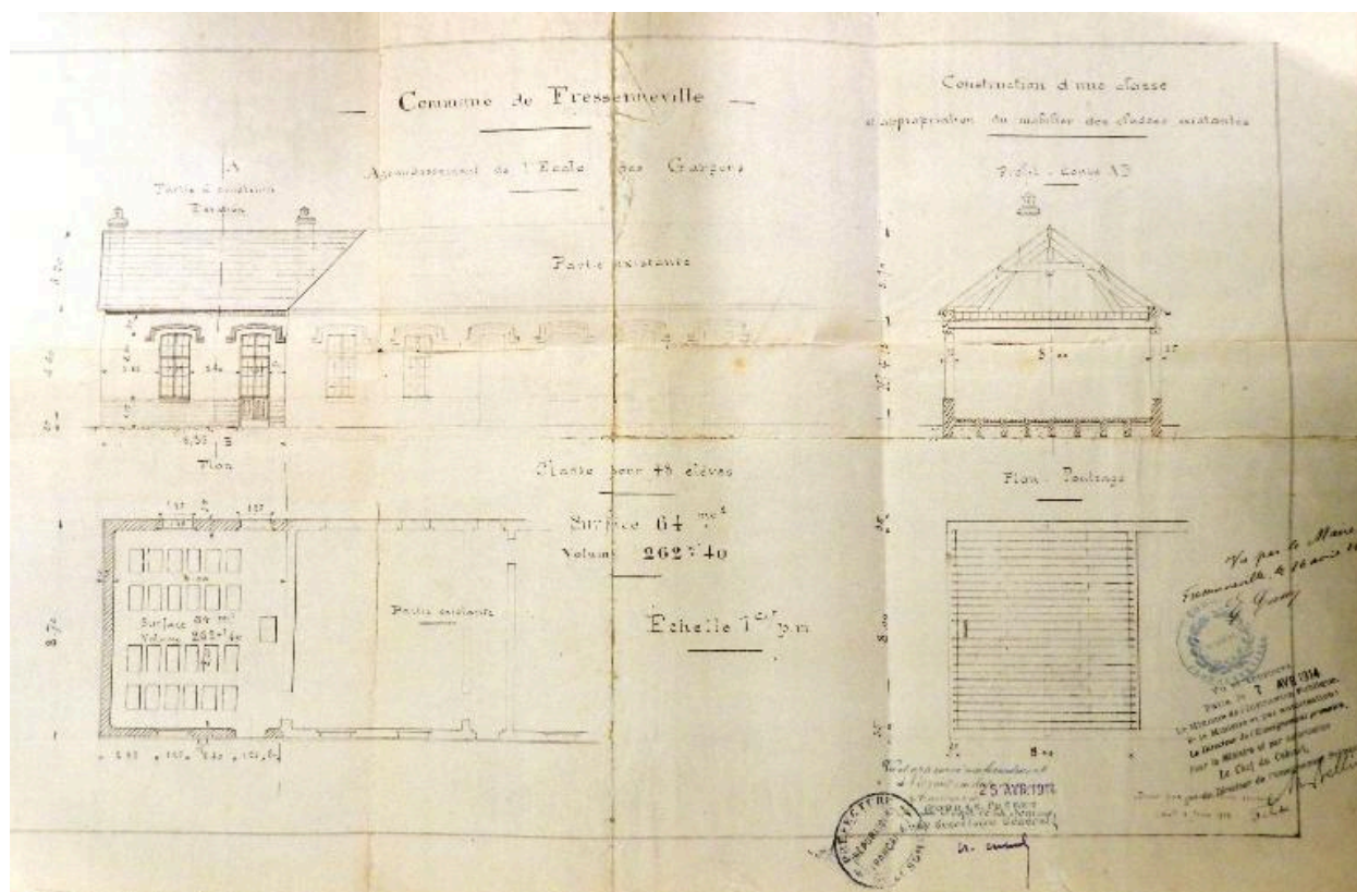
Fressenneville. Agrandissement de l'école de garçons. Plans, élévations et coupe par Chabot, 1912 (AD Somme ; 99 O 1871).
