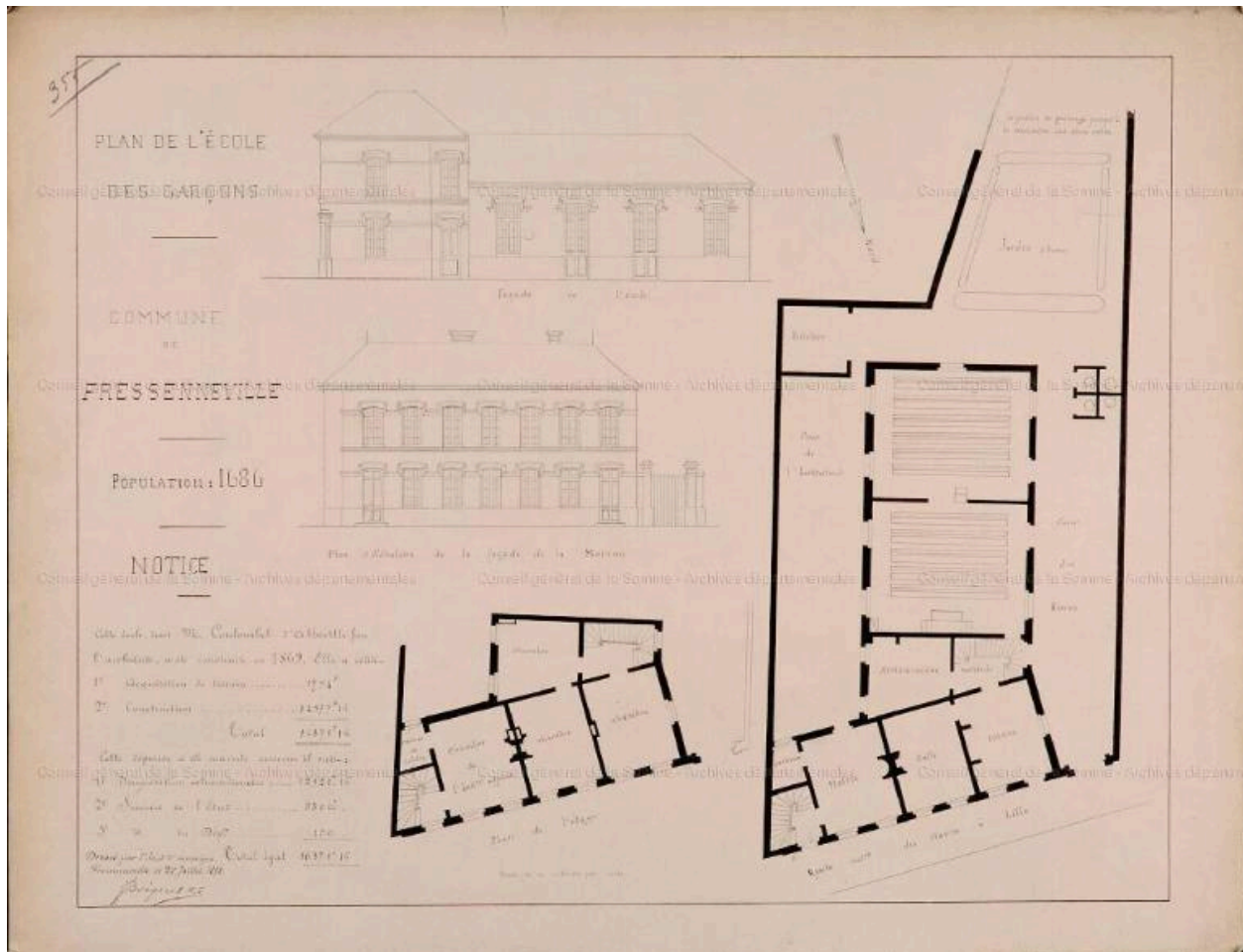
Commune de Fressenneville. Plan de l'école de garçons, 1878 (AD Somme ; 99T308 355/1).
