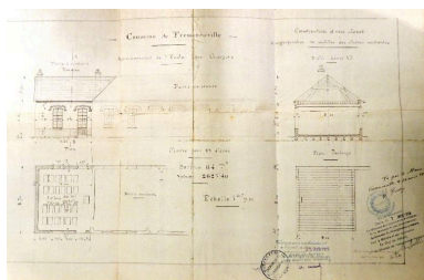
Fressenneville. Agrandissement de l'école de garçons. Plans,
