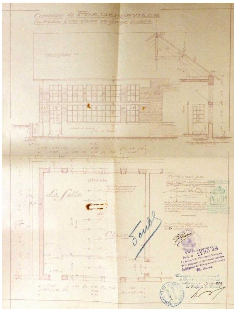
Commune de Fressenneville. Construction d'une classe au groupe scolaire. Élévation et plan, par André Echart architecte, 1935 (AD Somme ; 99 O 1871).
