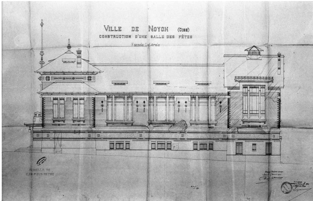
Elévation latérale, projet par C. Letrosne, 1903 (AD Oise ; série O).
