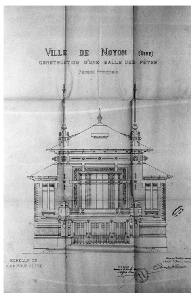
Élévation antérieure, projet par C. Letrosne, 1903 (AD Oise ; série O). Phot. Jean-Michel Périn IVR22_19846000359XB
