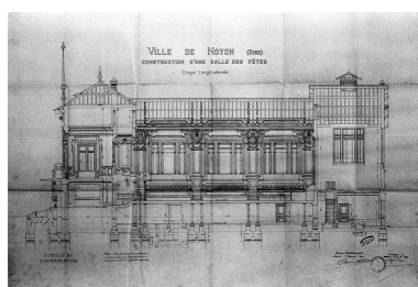
Coupe longitudinale, projet par C. Letrosne, 1903 (AD Oise ; série O). Phot. Jean-Michel Périn IVR22_19846000360XB
