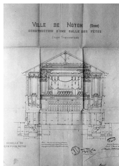
Coupe transversale, projet par C. Letrosne, 1903 (AD Oise ; série O). Phot. Jean-Michel Périn IVR22_19846000337XB
