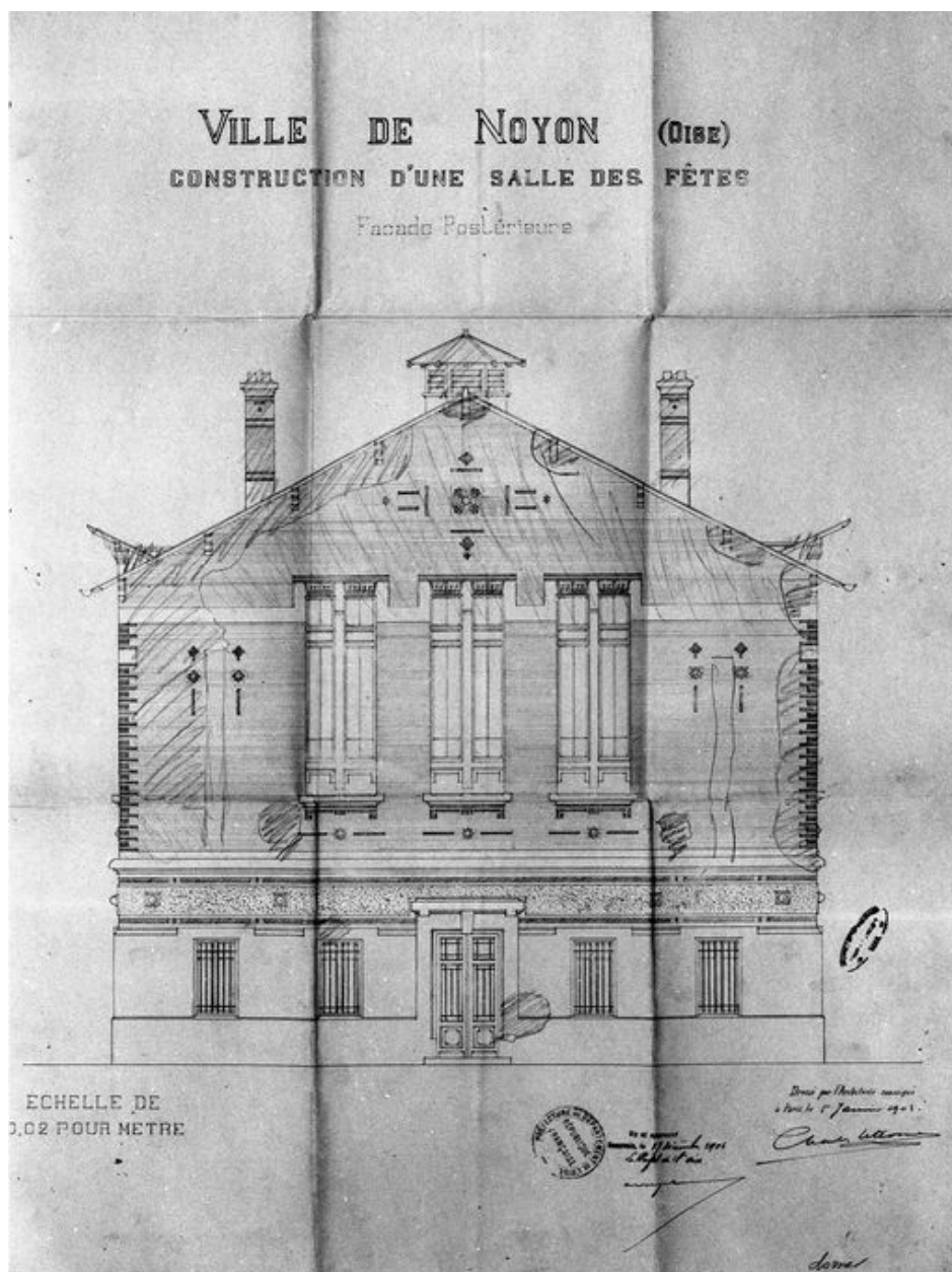
Elévation postérieure, projet par C. Letrosne, 1903 (AD Oise ; série O).
