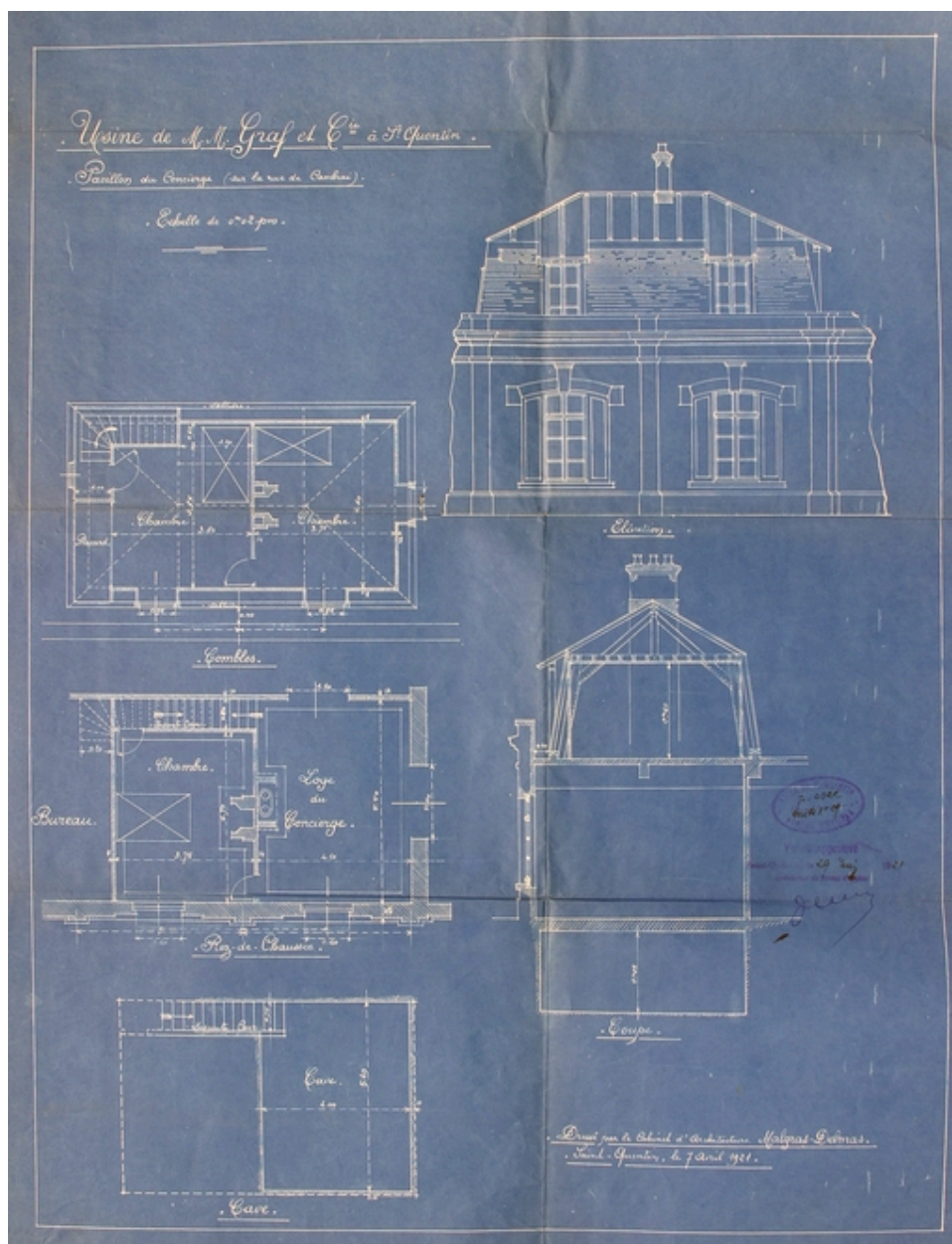
Plans de la concoergerie, par Malgras-Delmas, 1921 (AC Saint-Quentin).
