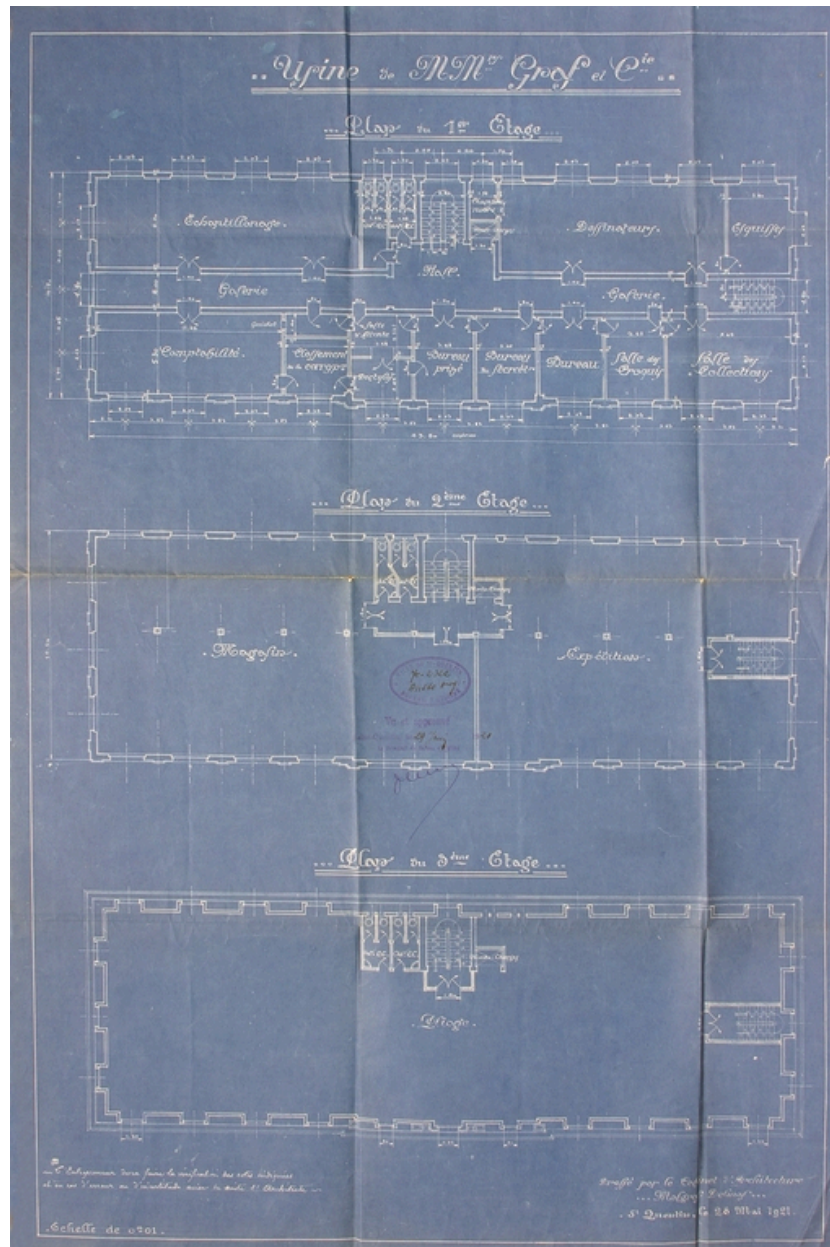
Plan par niveau de la maison de commerce projetée, par Malgras-Delmas, 1921 (AC Saint-Quentin).
