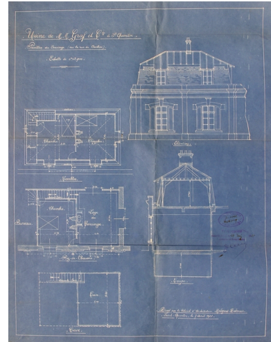
Plans de la conciergerie, par Malgras-Delmas, 1921 (AC Saint-Quentin). Repro. Frédéric Pillet IVR22_20060205722NUCAB
