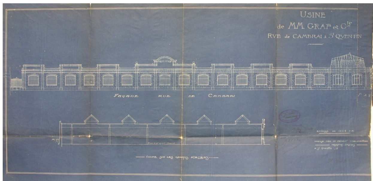
Projet de reconstruction de l'usine, façade antérieure des ateliers, par Malgras-Delmas, vers 1920 (AC Saint-Quentin).
