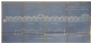
Projet de reconstruction de l'usine, façade antérieure des ateliers, par Malgras-Delmas, vers 1920 (AC Saint-Quentin). Repro. Frédéric Pillet IVR22_20060205719NUCAB
