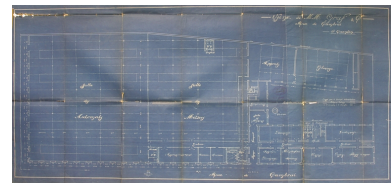
Projet de reconstruction de l'usine, plan du rez-de-chaussée, par Malgras-Delmas, 1920 (AC Saint-Quentin). Repro. Frédéric Pillet IVR22_20060205717NUCAB
