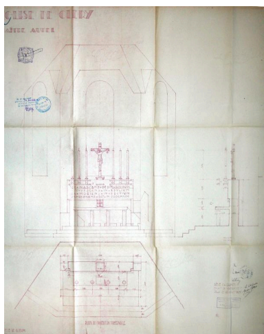
Maître-autel (plan, coupe et élévation au niveau du tabernacle), Jacques Debat-Ponsan (architecte), 24 juillet 1931 (AD Somme ; 99 O 1182). Phot. Gilles-Henri Bailly (reproduction) IVR22_20158005526NUCA
