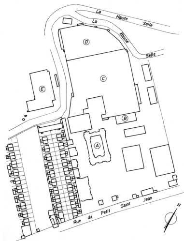
Schéma de situation : A. Etablissement thermal, B. Salle des machines, C. D. Ateliers de filature, E. Ateliers de tissage. Dess. Monnehay-Vulliet Marie-Laure , Autr. Stéphane Gonet IVR32_20168000833NUD
