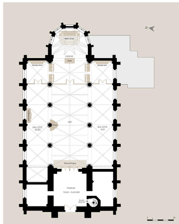
Plan de l'église Notre-Dame-de-l'Assomption. Dess. Eddy Stein IVR32_20265900002NUDA
