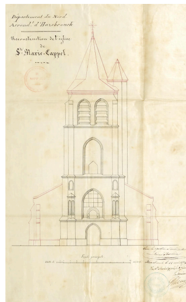
Reconstruction de l'église de Sainte-Marie-Cappel - façade principale. Dressé par l'architecte LÉONARD BARBIER le 28 mai 1874 (AD Nord 2 O 535 / 16). Repro. Delphine Volto Jourdan IVR32_20255900573NUCA
