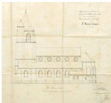
Reconstruction de l'église de Sainte-Marie-Cappel - élévation latérale. Dressé par l'architecte LÉONARD BARBIER le 28 mai 1874 (AD Nord 2 O 535 / 16). Repro. Delphine Volto Jourdan IVR32_20255900574NUCA
