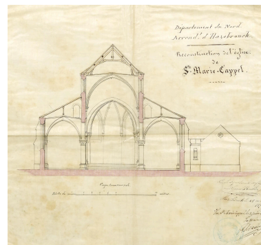
Reconstruction de l'église de Sainte-Marie-Cappel - coupe transversale. Plan dressé par l'architecte LÉONARD BARBIER le 28 mai 1874 (AD Nord 2 O 535 / 16). Repro. Delphine Volto Jourdan IVR32_20255900576NUCA
