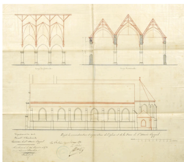
Reconstruction de l'église de Sainte-Marie-Cappel - différentes coupes
