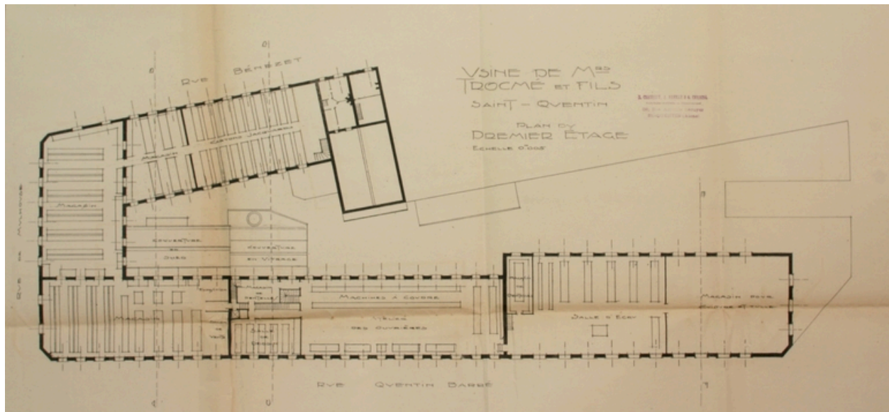
Plan du premier étage de l'usine Trocmé à la veille de la Première Guerre mondiale, dressé après 1919 par Chauquet, Navile et Christol (AD Aisne).
