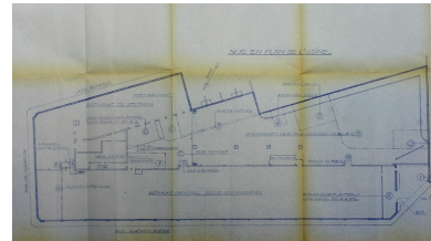
Imprimerie Peter - Saint-Quentin - Aménagement de l'usine, plan d'ensemble et repérage, par Chleq Froté et Cie, 1964 (AC Saint-Quentin). Phot. Pillet Frédéric IVR22_20040200642NUCAB
