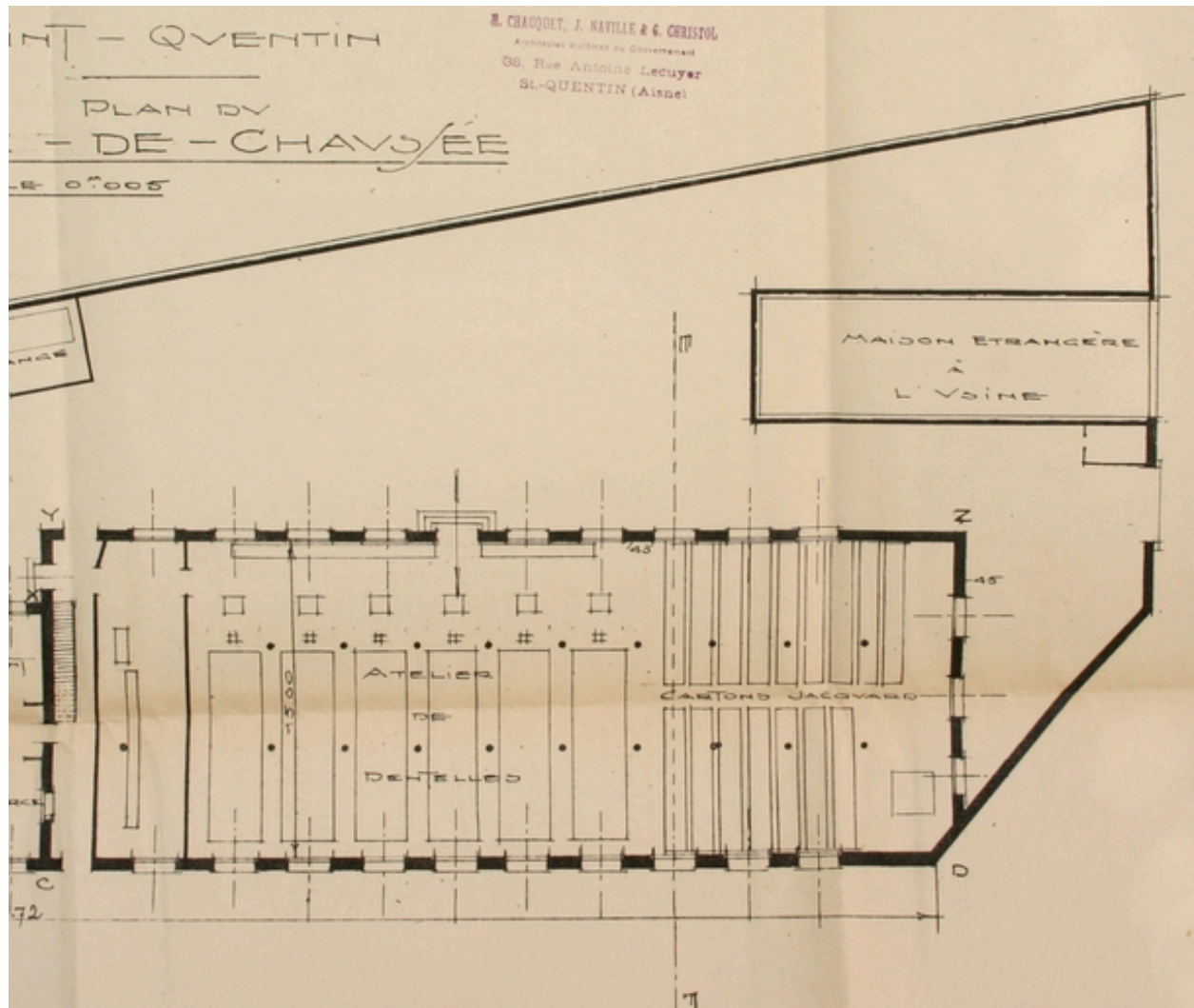
Plan du rez-de-chaussée de l'usine Trocmé à la veille de la Première Guerre mondiale, dressé après 1919 par Chauquet, Naville et Christol. Détail de l'atelier de dentelle (AD Aisne).
