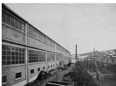
Les ateliers en cours de reconstruction, 1920 (Le Monde Illustré). Phot. Pillet Frédéric IVR22_20040200588NUCAB
