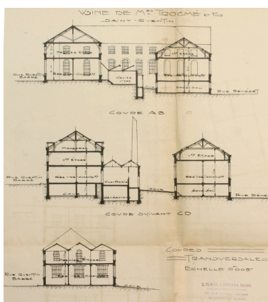
Coupes transversales de l'usine Trocmé à la veille de la Première Guerre mondiale, dressées après 1919 par Chauquet, Navile et Christol (AD Aisne). Phot. Pillet Frédéric IVR22_20040200581NUCAB
