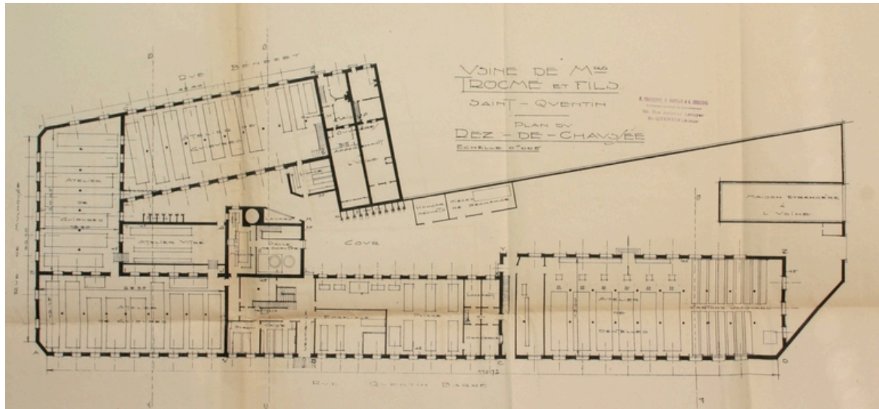
Plan du rez-de-chaussée de l'usine Trocmé à la veille de la Première Guerre mondiale dressé après 1919 par Chauquet, Navile et Christol (AD Aisne).
