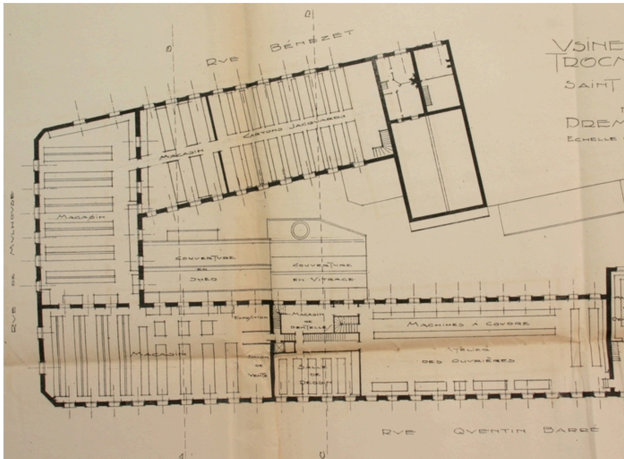
Plan du premier étage de l'usine Trocmé à la veille de la Première Guerre mondiale dressé après 1919 par Chauquet, Navile et Christol. Détail des magasins, de la salle de dessin, de l'atelier de couture (AD Aisne).
