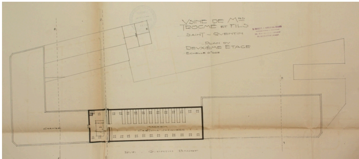
Plan du deuxième étage de l'usine Trocmé à la veille de la Première Guerre mondiale, dressé après 1919 par Chauquet, Navile et Christol (AD Aisne).
