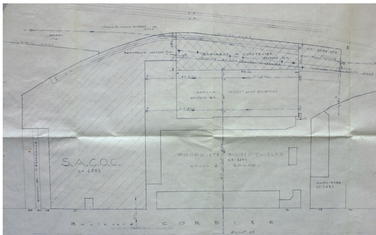
Plan masse de la cartonnerie en 1977 (AC Saint-Quentin).
