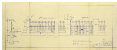
Relevé en élévation d'un projet de clôture autour du cimetière de Bavinchove, 5 avril 1833 (AD Nord : 2 O 54 / 22). IVR32_20255900590NUCA
