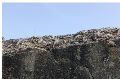
Partie est, détail du béton et des fers Phot. Jean-Marc Ramette IVR31_20145904860NUCA
