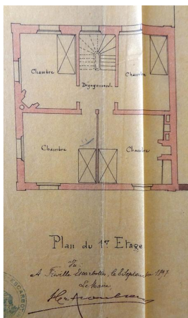
Projet de construction d'un bureau de poste. Plan du 1er étage, A. Marchand architecte, 1898 (AD Somme ; 99 O 1904). Phot. Frédéric-Nicolas Kocourek (reproduction) IVR22_20148005098NUC2A
