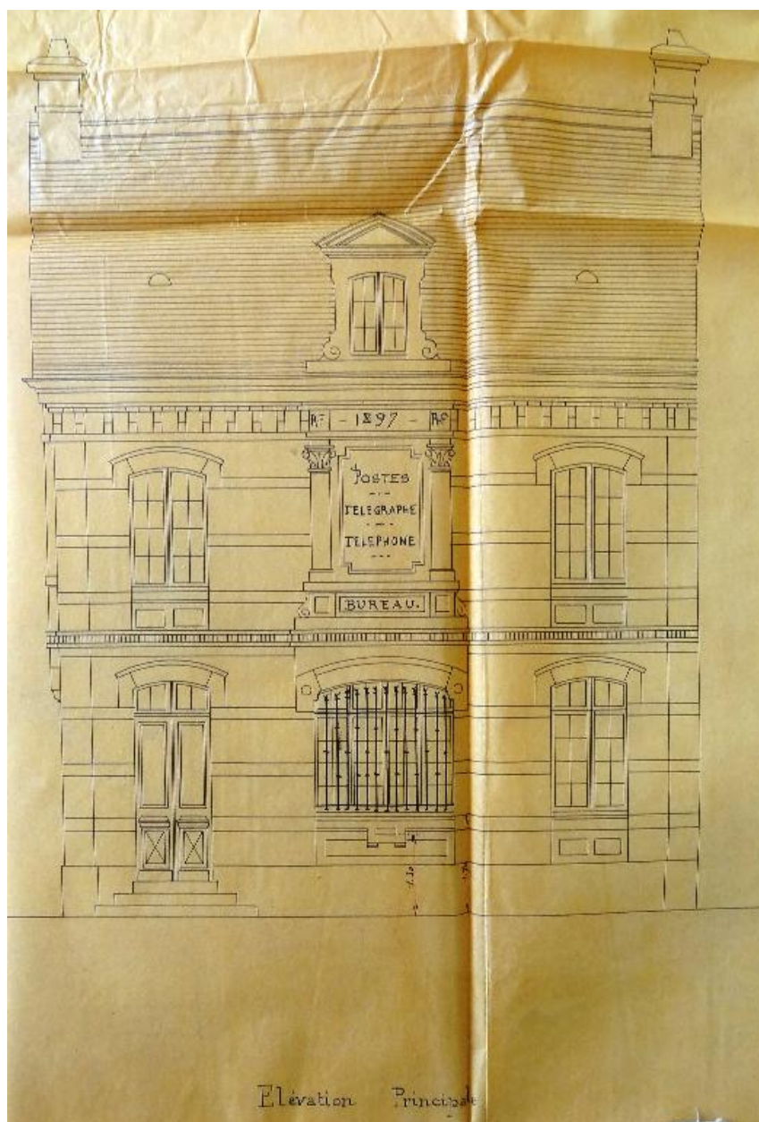
Projet de construction d'un bureau de poste. Élévation principale, A. Marchand architecte, 1898 (AD Somme ; 99 O 1904).
