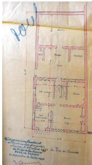
Projet de construction d'un bureau de poste. Plan du rez-de-chaussée, A. Marchand architecte, 1898 (AD Somme ; 99 O 1904). Phot. Frédéric-Nicolas Kocourek (reproduction) IVR22_20148005097NUC2A
