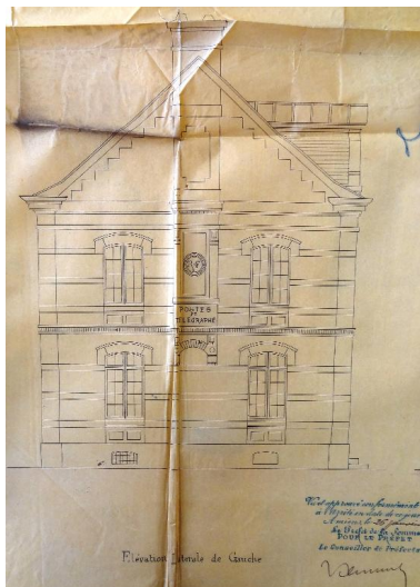
Projet de construction d'un bureau de poste. Élévation latérale de gauche, A. Marchand architecte, 1898 (AD Somme ; 99 O 1904). Phot. Frédéric-Nicolas Kocourek IVR22_20148005173NUC2A
