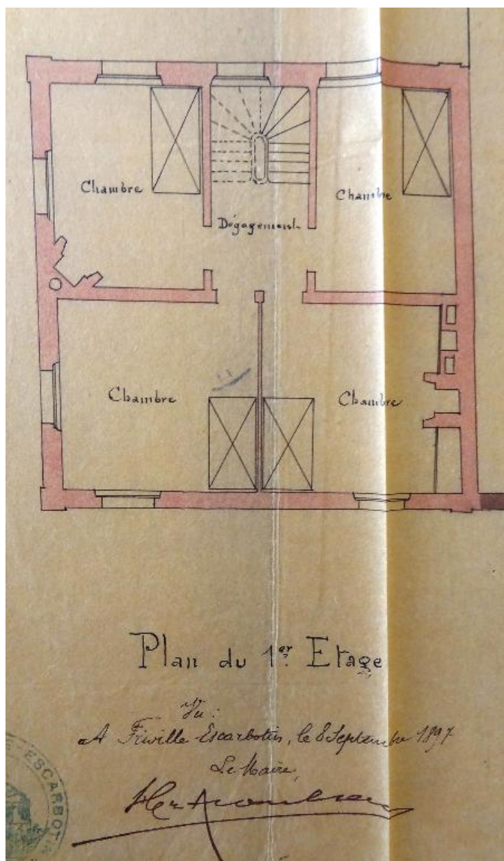
Projet de construction d'un bureau de poste. Plan du 1er étage, A. Marchand architecte, 1898 (AD Somme ; 99 O 1904).
