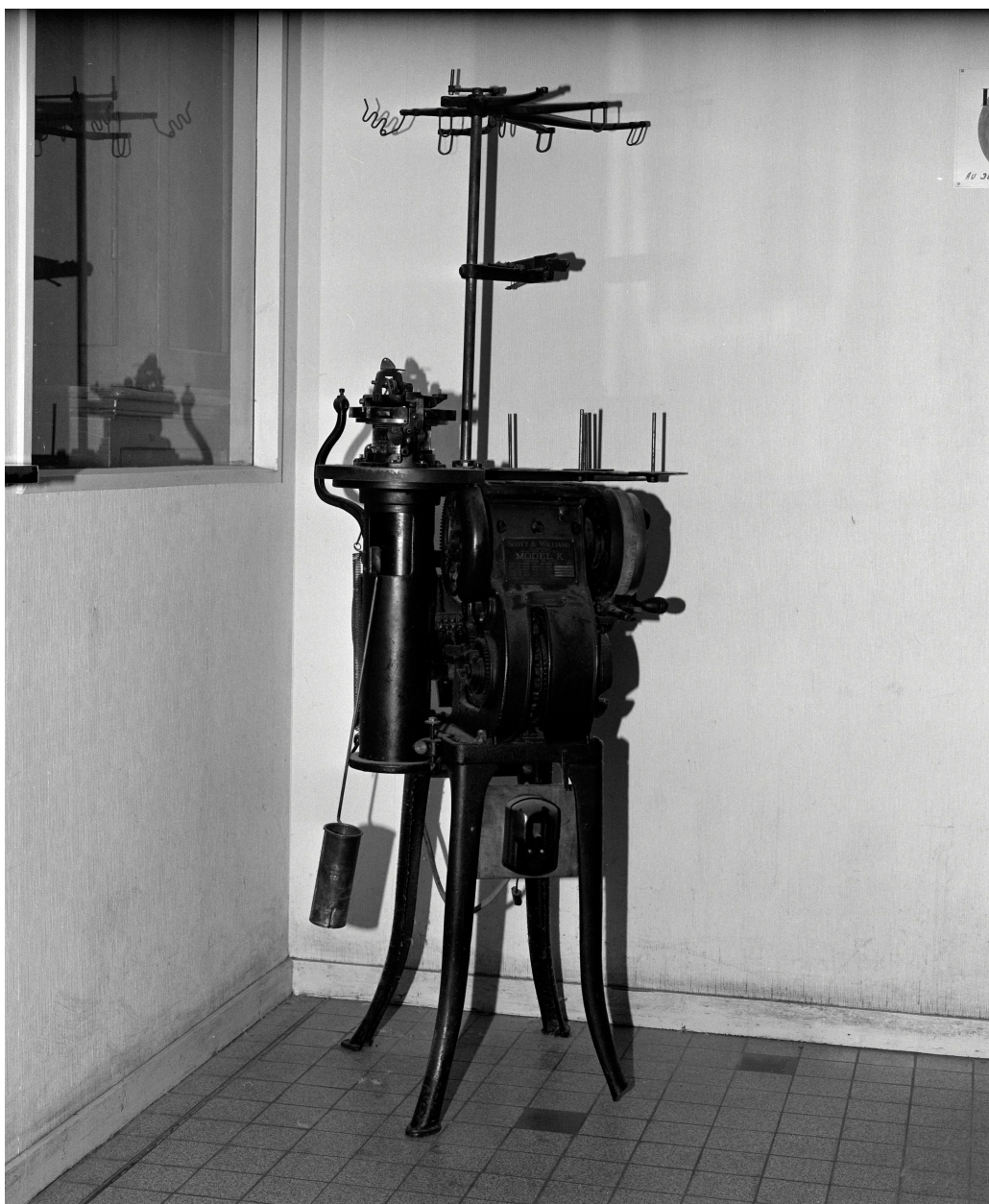
Bureaux. Tricoteuse Scott & Williams.
