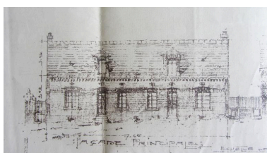
Façade principale d'une maison ouvrière, rue Alfred-Maguin, 20 novembre 1920 (AD Aisne ; 15 R 772). Phot. Fournier Bertrand (reproduction) IVR32_20160205089NUC2A
