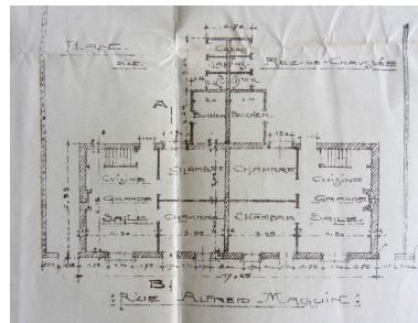
Plan du rez-de-chaussée d'une des maisons ouvrières, rue Alfred-Maguin, 20 novembre 1920 (AD Aisne ; 15 R 772). Phot. Fournier Bertrand (reproduction) IVR32_20160205087NUC2A
