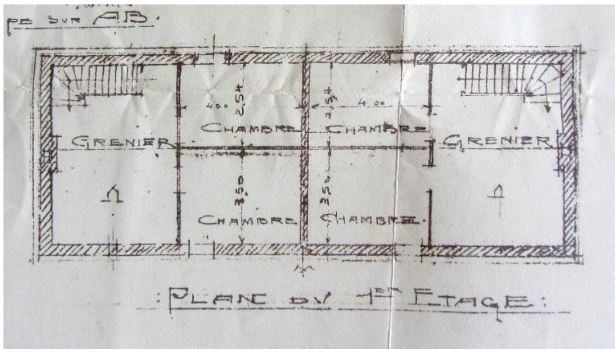
Plan de l'étage d'une des maisons ouvrières, rue Alfred-Maguin, 20 novembre 1920 (AD Aisne ; 15 R 772).
