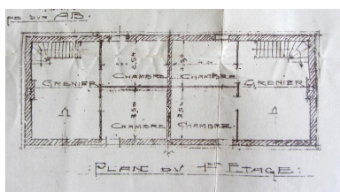
Plan de l'étage d'une des maisons ouvrières, rue Alfred-Maguin, 20 novembre 1920 (AD Aisne ; 15 R 772). Phot. Fournier Bertrand (reproduction) IVR32_20160205088NUC2A
