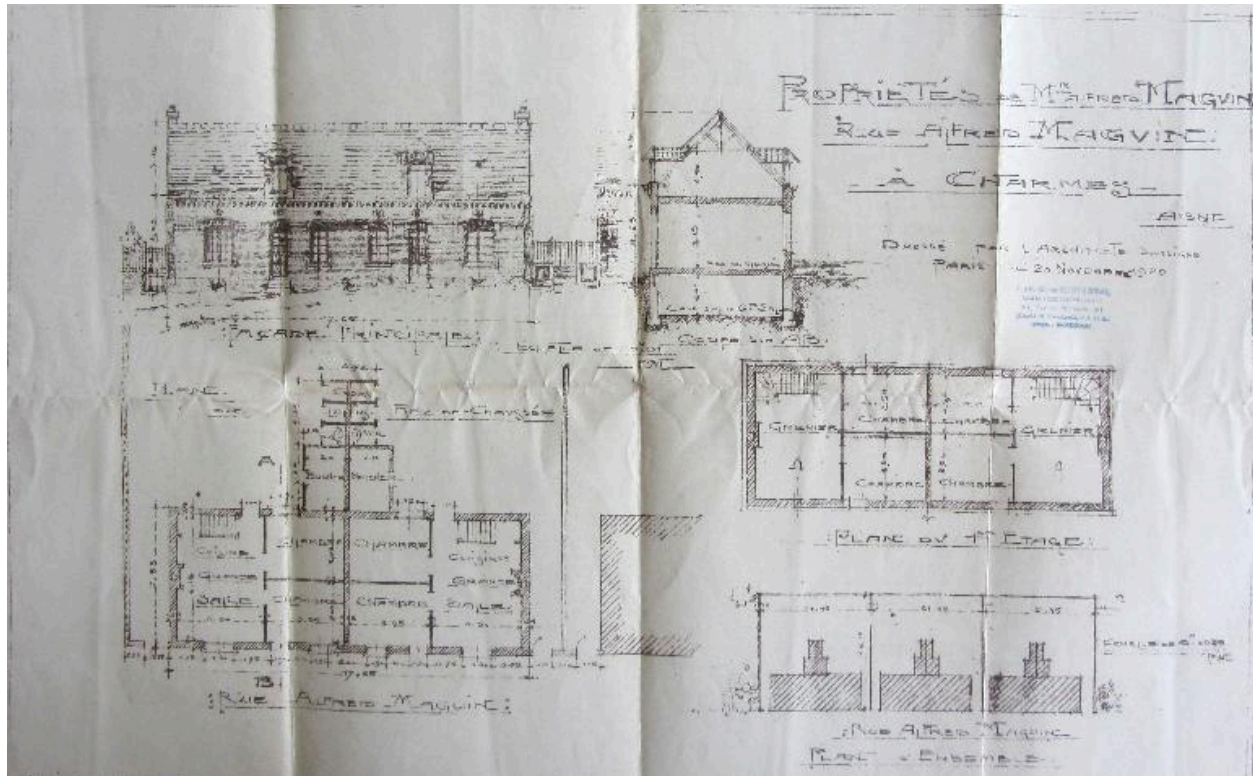
Plans coupes et élévations des trois maisons ouvrières endommagées rue Alfred-Maguin, dressés par J. de Montarnal, 20 novembre 1920 (AD Aisne ; 15 R 772).
