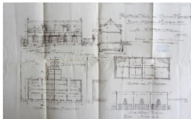
Plans coupes et élévations des trois maisons ouvrières endommagées rue Alfred-Maguin, dressés par J. de Montarnal, 20 novembre 1920 (AD Aisne ; 15 R 772). Phot. Fournier Bertrand (reproduction) IVR32_20160205090NUC2A
