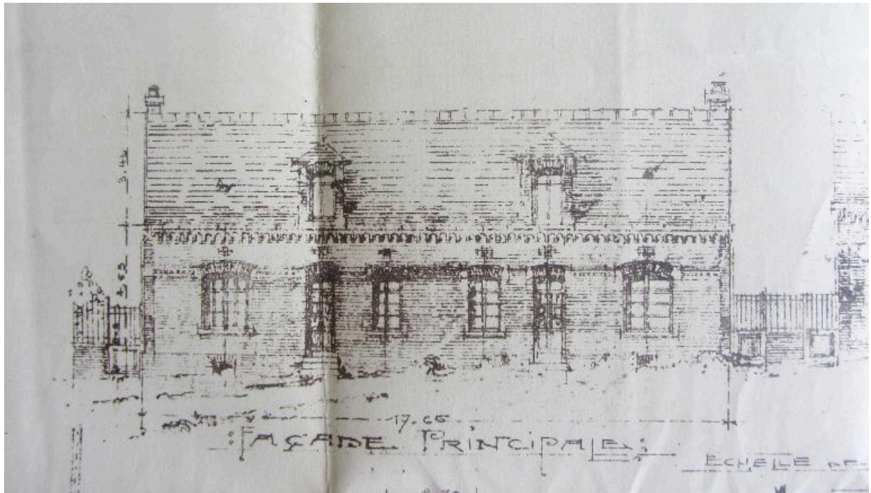
Façade principale d'une maison ouvrière, rue Alfred-Maguin, 20 novembre 1920 (AD Aisne ; 15 R 772).
