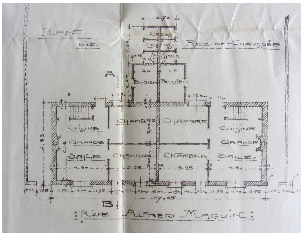
Plan du rez-de-chaussée d'une des maisons ouvrières, rue Alfred-Maguin, 20 novembre 1920 (AD Aisne ; 15 R 772).
