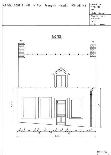
Façade, élévation.
