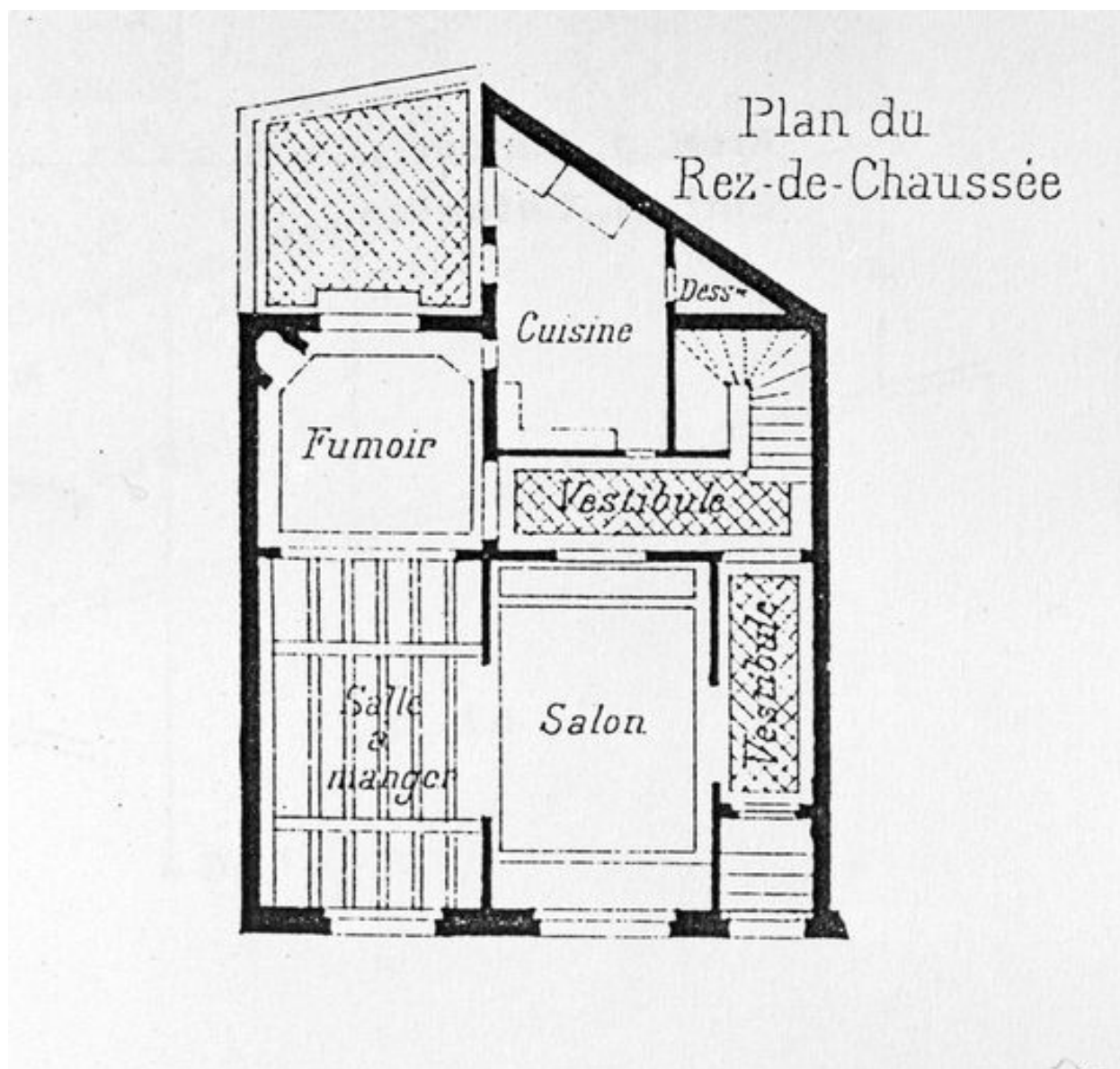
Plan du rez-de-chaussée de la Villa Bon-Temps, d'après Ernest Bertrand architecte. In : Villas et cottages des bords de la mer. Charles Schmid, [ca 1910].
