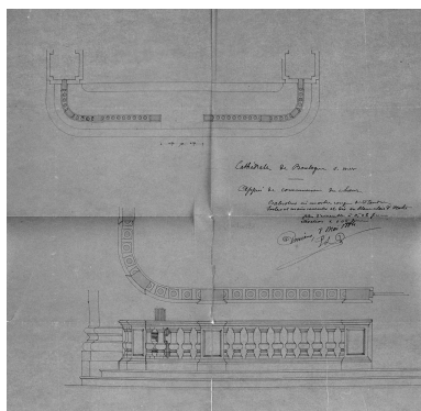
Plan, élévation, signé Duthoit, daté 1884 (AD Pas- de-Calais, 9 J 20 P 100). Repro. Olivier Marlard IVR31_19886200535X
