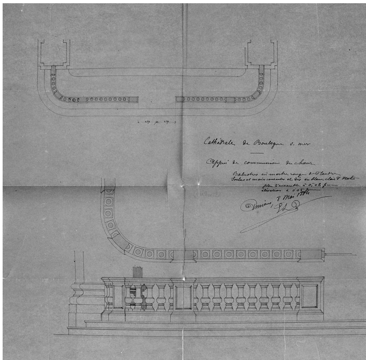
Plan, élévation, signé Duthoit, daté 1884 (AD Pas-de-Calais, 9 J 20 P 100).
