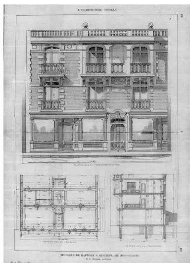
Plan et élévation dans la revue L'architecture usuelle, 1926, pp. 108, 109. Phot. Bouvet Hubert IVR31_20106201152NUCB
