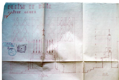
Coupe et élévation du maître-autel, Jacques Debat-Ponsan (architecte), 16 juillet 1931 (AD Somme ; 99 O 902). Repro. Gilles-Henri Bailly IVR22_20158005492NUCA
