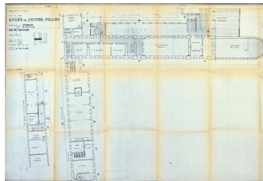
Plan du rez-de-chaussée montrant la destination des différents espaces, signé Coasnes, novembre 1962. (AC Douai, 676W8) Phot. Pierre Thibaut IVR32_20225900418NUCA
