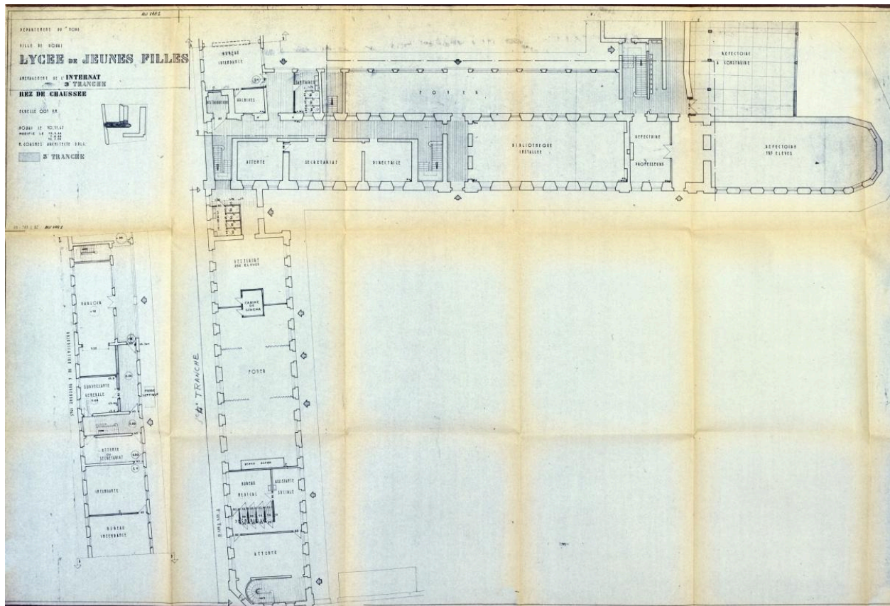
Plan du rez-de-chaussée montrant la destination des différents espaces, signé Coasnes, novembre 1962. (AC Douai, 676W8)
