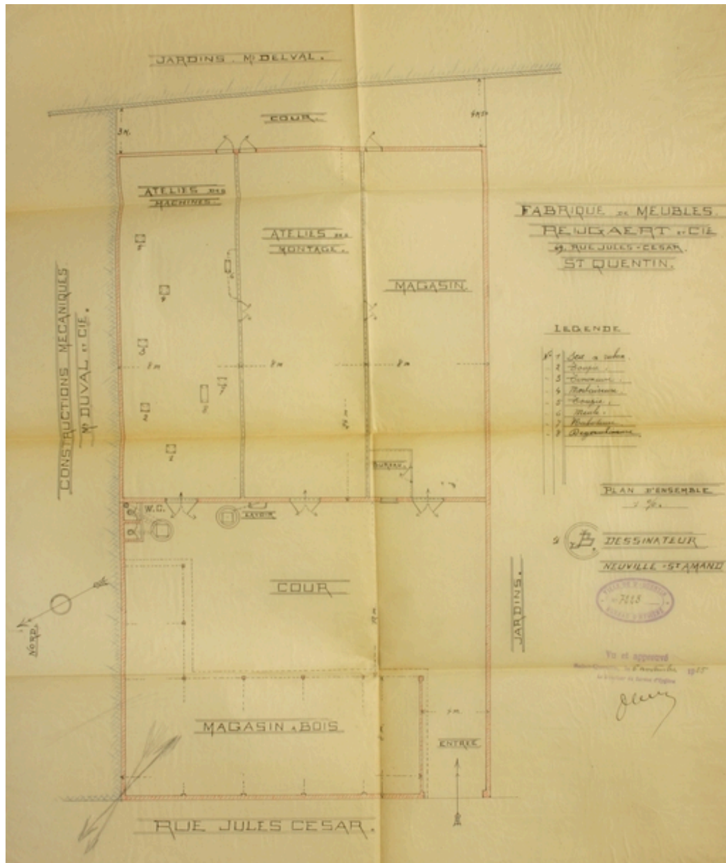
Plan d'ensemble de l'usine en 1925 (AC Saint-Quentin).
