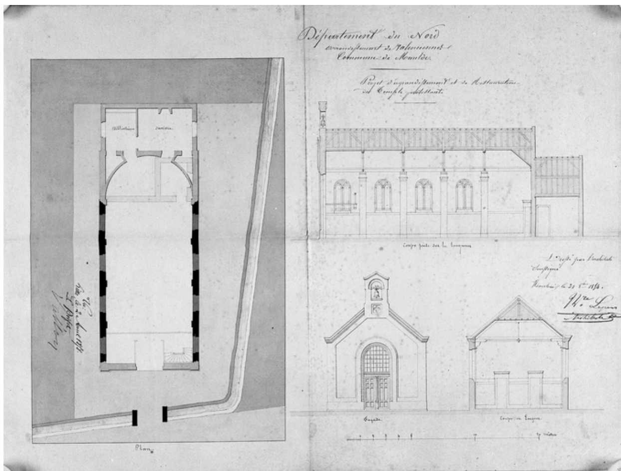
Projet d'agrandissement et de restauration (plan, élévation antérieure, coupes), Lepers architecte, 1854 (AD Nord : 7 V/21).
