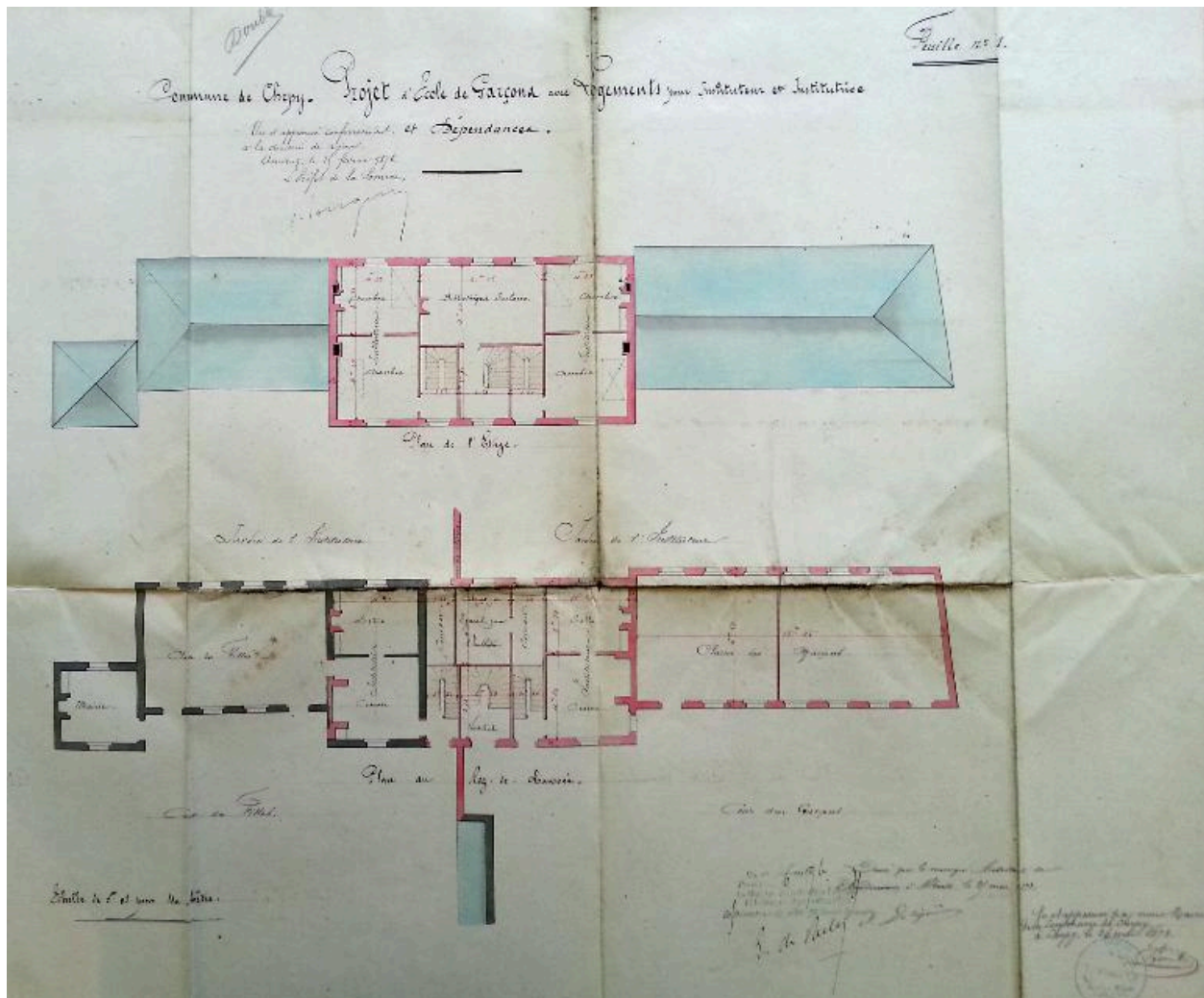
Plans des étages, dressés par l'architecte Delignères, en 1873 (AD Somme ; 99 O 1145).
