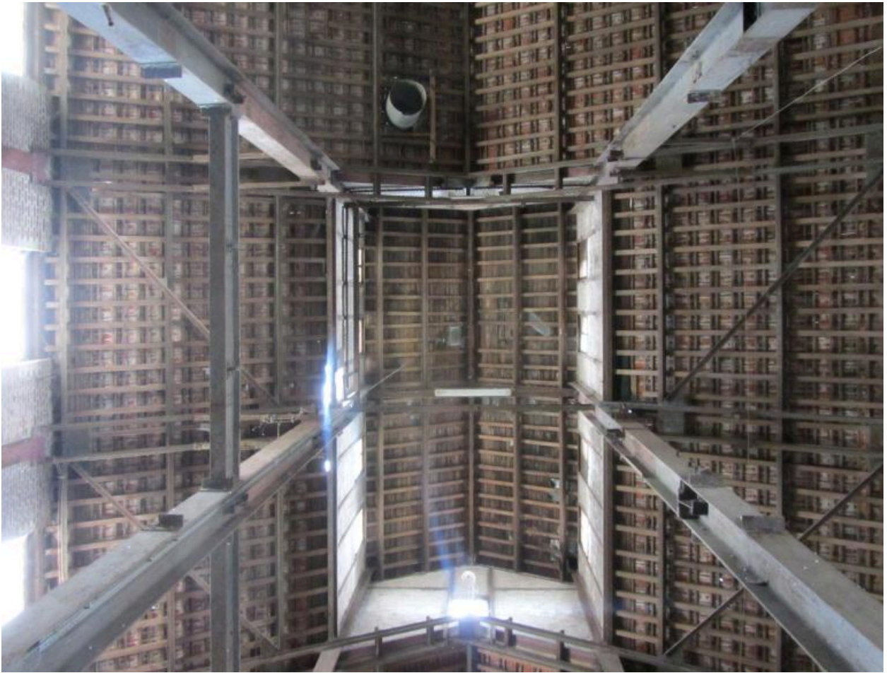
Vue intérieure de la charpente métallique de l'atelier principal de la râperie.
