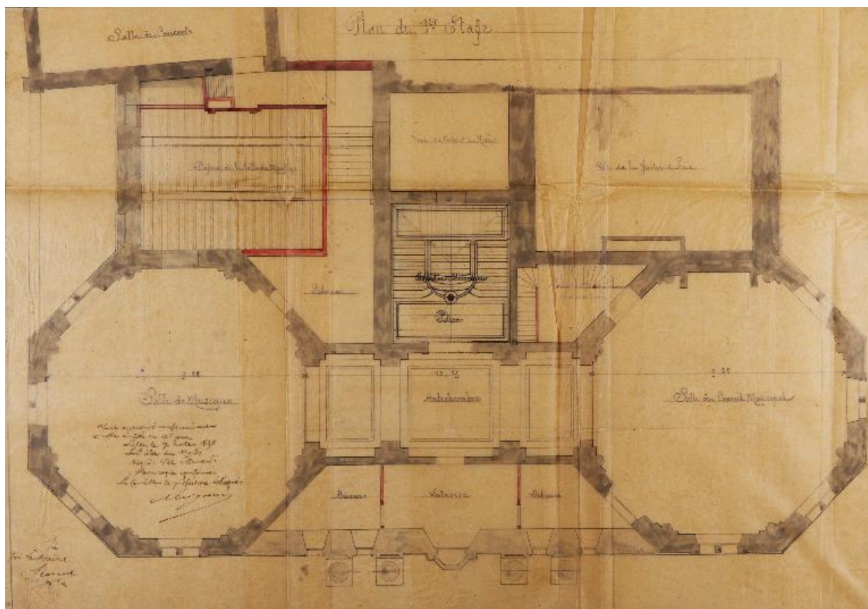
Plan du premier étage avec l'escalier d'honneur, Vandembuleke (?) architecte, 1890 (AD Nord, Série 2O 525/87).
