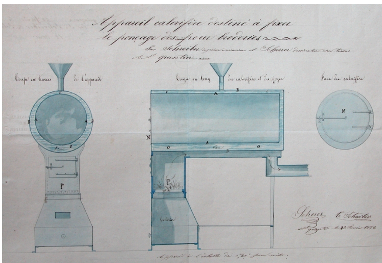
Appareil calorifique destiné à fixer le ponçage des dessins pour broderies. Théodore Schreiber et Adelbert Scherer, 1852 (INPI).
