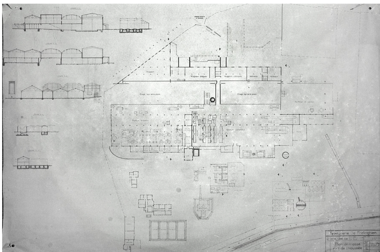
Teinturerie de Frelinghien (TDF). Plan masse du rez-de-chaussée, 1924 (AD Nord ; M41712466).
